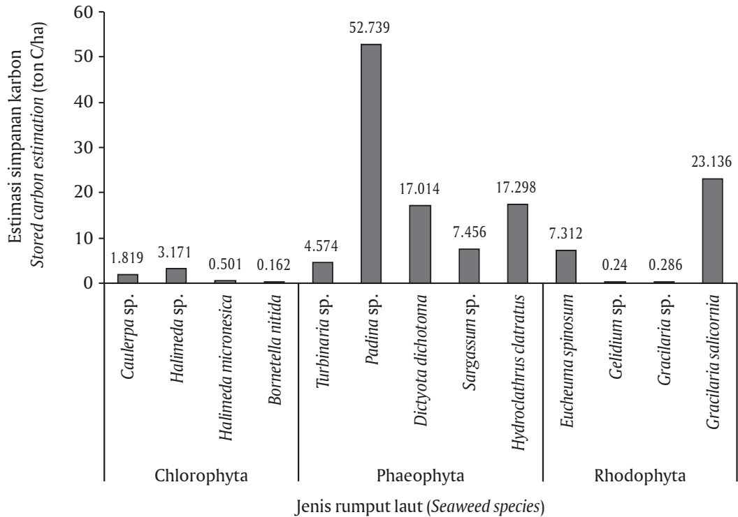
Gambar 7. Estimasi simpanan karbon beberapa jenis rumput laut alam berdasarkan luas tutupan di kawasan rata-rata terumbu Labuhanbua, Kabupaten Sumbawa, Nusa Tenggara Barat
