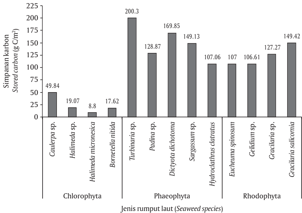
Gambar 6. Variasi simpanan karbon beberapa jenis rumput laut alam di kawasan rata-rata terumbu Labuhanbua, Kabupaten Sumbawa, Nusa Tenggara Barat
