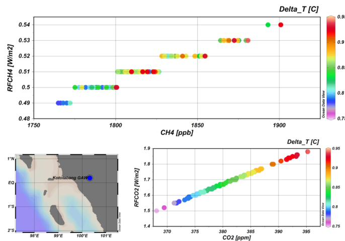
Gambar 10. Hubungan antara Radiative Forcing CH 4 dengan Selisih Suhu Udara pada 2004 - 2013.
