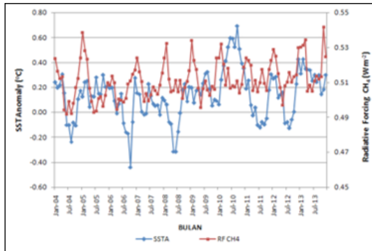
Gambar 13. Perbandingan Permukaan Laut Anomali Indonesia dan Radiative Forcing Metana di Bukit Kototabang.
