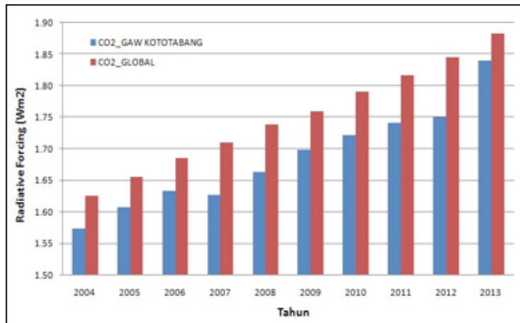
Gambar 4. KRF CO 2 di GAW Bukit Kototabang dan Rerata Global.
