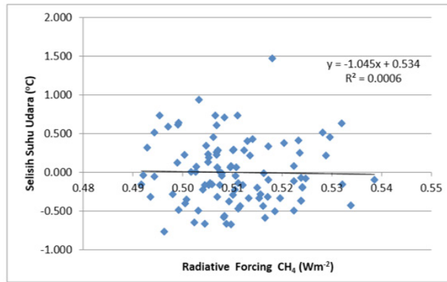
Gambar 9. Hubungan antara Radiative Forcing CH 4 dengan Selisih Suhu Udara pada 2004 - 2013.
