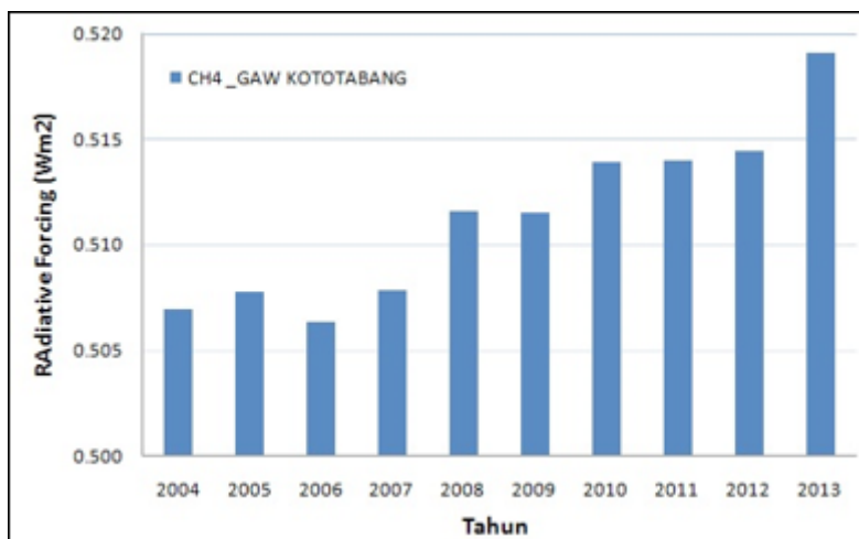
Gambar 5. RF CH 4 di GAW Bukit Kototabang.
