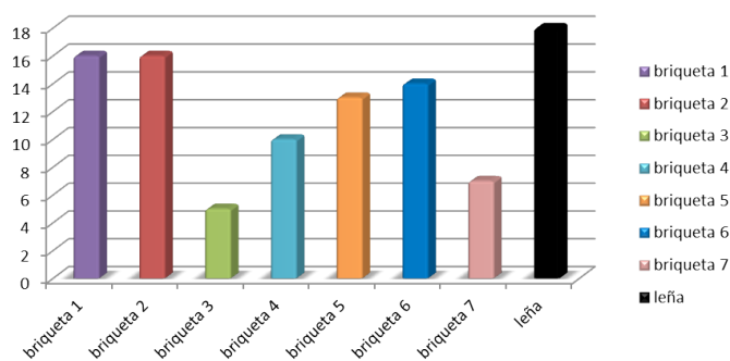
Gráfica 1: Tiempo de ebullicion del agua (minutos)
