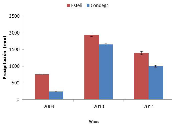
Fig.3: Acumulado de las precipitaciones registrados en las estaciones del Limón en Estelí y Condega. Las barras representan la sumatoria de la lluvia caída en los doce meses de cada año.
