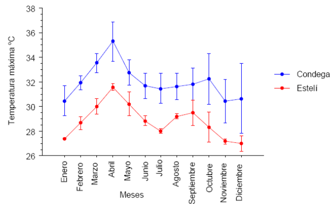
Fig. 1: Comportamiento de las temperaturas máximas promedio en los años 2009 al 2011, en los municipios de Condega y Estelí.
