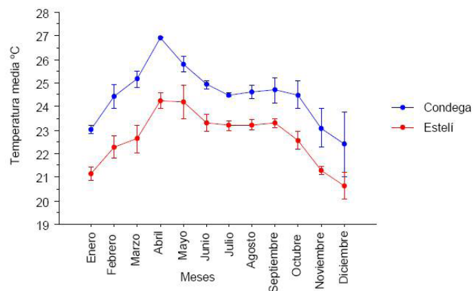
Fig. 3: Comportamiento de las temperaturas medias en los años 2009 al 2011.
