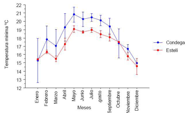
Fig. 2: Comportamiento de las temperaturas mínimas promedio en los años 2009 al 2011, en los municipios de Condega y Estelí.
