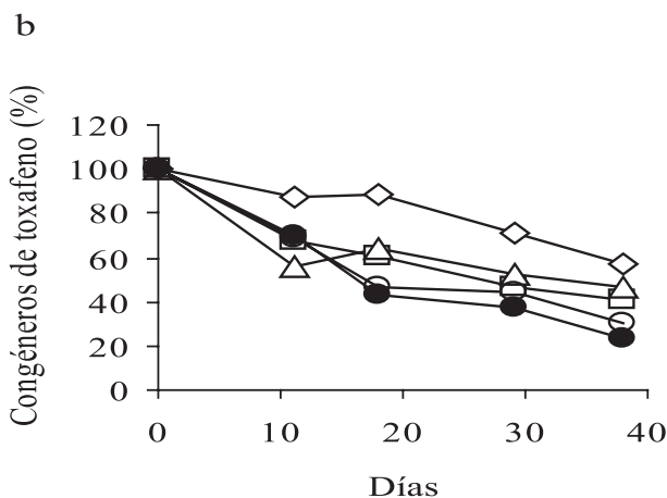
Ilustración 2. Degradación del toxafeno por la especie Bjerkandera sp BOL13 con virutas de madera (b) y (c) melazas de caña. Los isómeros son representados por símbolos: P11
