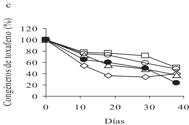
Ilustración 3. Degradación del toxafeno por la especie Bjerkandera sp BOL13 con melazas de caña (c). Los isómeros son representados por símbolos: P11 representado por rombos, P32 por cuadrados, P31 por triángulos, P50 por círculos abiertos y P69 por círculos negros. La degradación del toxafeno fue seguida durante 38 días de incubación. Los valores graficados representan los valores medios de los datos obtenidos de los lotes de cultivos realizados por duplicado.
