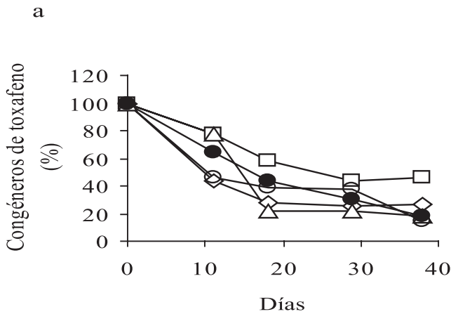
Ilustración 1. Degradación del toxafeno por la especie Bjerkandera sp BOL13 con cáscara de trigo (a). Los isómeros son representados por símbolos: P11 representado por rombos, P32 por cuadrados, P31 por triángulos, P50 por círculos abiertos y P69 por círculos negros. La degradación del toxafeno fue seguida durante 38 días de incubación. Los valores graficados representan los valores medios de los datos obtenidos de los lotes de cultivos realizados por duplicado.
