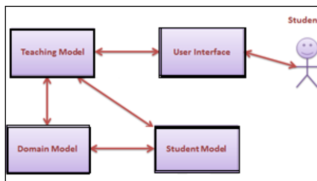
Fig 1: DES-Tutor Architecture.
