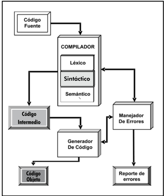
Diagrama 1. Proceso de compilación
