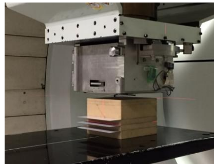
図4 陽子線治療装置でのファントム実験
