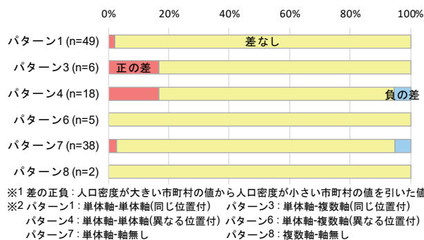
図-7 市町村間における差の有無(車線数)
