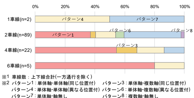
図-9 人口密度が大きい市町村からの車線数と整合性
