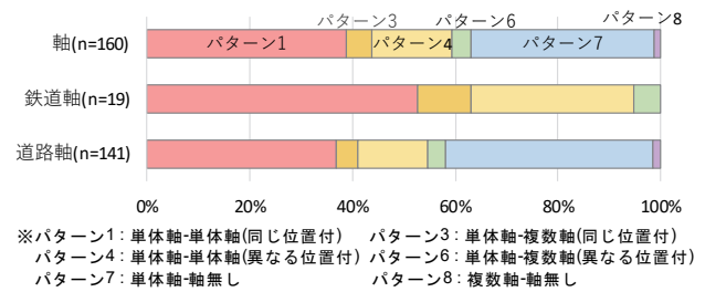
図-2 軸パターン別にみた市町村間の整合性
