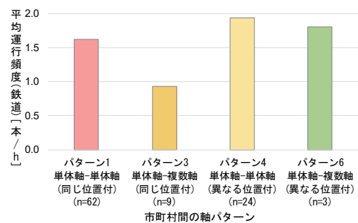
図-4 市町村間での軸パターン別に見た鉄道の平均運行頻度
