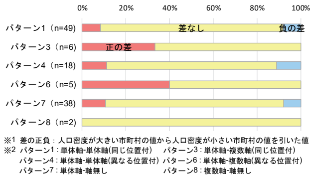
図-6 市町村間における差の有無(道路交通量)
