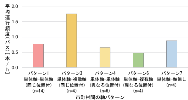
図-5 市町村間での軸パターン別に見たバスの平均運行頻度
