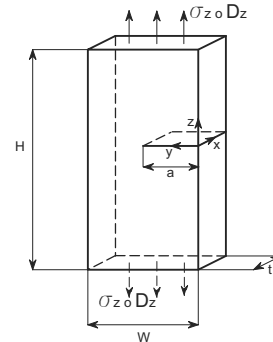
Figura 1. Esquema del problema de grieta recta de borde.
