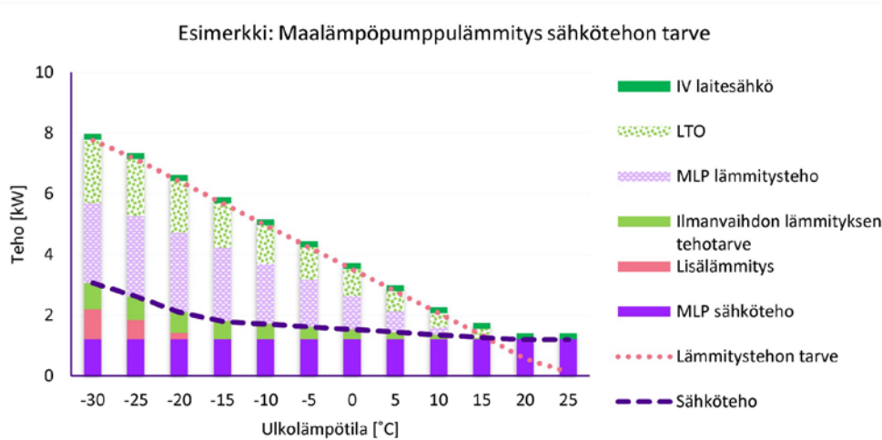
Kuva 5.10 Esimerkki maalämpöratkaisun sähkötehon tarpeesta (Esimerkkikohde A_{\text{netto}} 125 m 2 )
