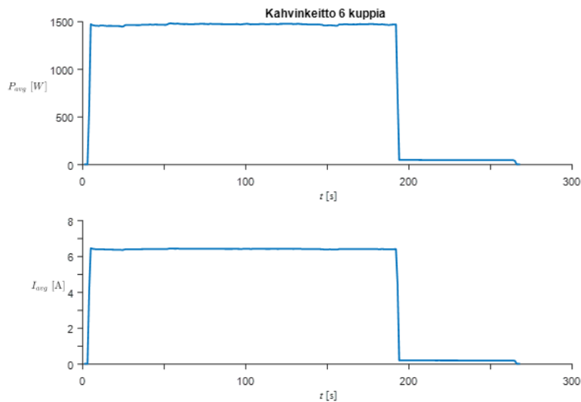
Kuva 0.1 Kahvinkeitin tehoprofiili
