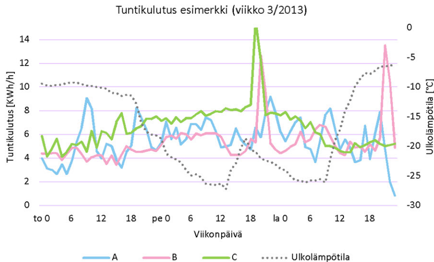
Kuva 2.2 Esimerkki kolmen pientalon energiakulutuspöytästä verkon huippukulutusaikana. Tuntimittaus.
