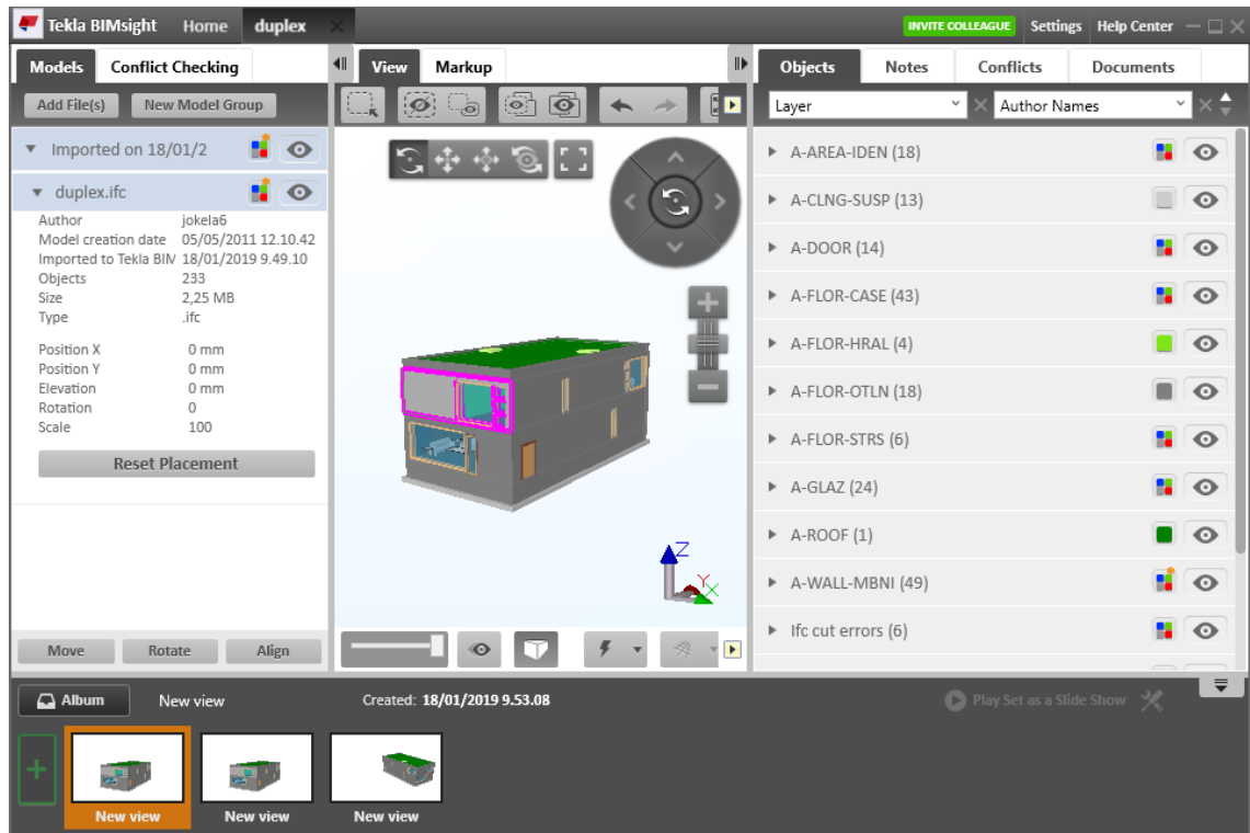
Kuva 5. Tekla BIMsight
