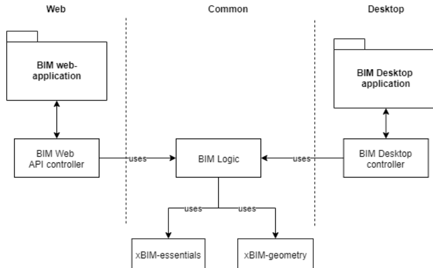
Kuva 17. Yhteinen BIM-logiikka
