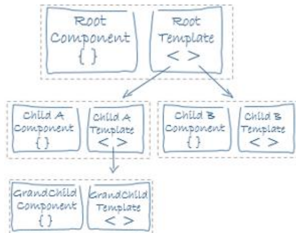
Kuva 11. Angularin näkymähierarkia [16]
