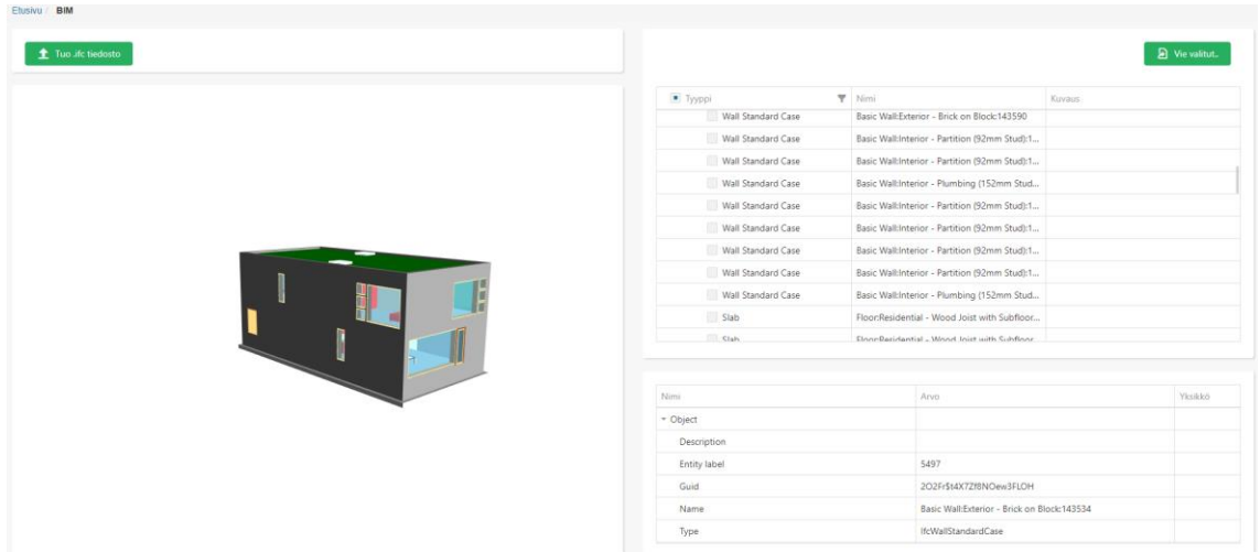
Kuva 30. Verkkopohjainen BIM-työkalu
