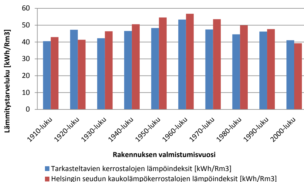
Kuva 3.8. Kerrostalojen lämmitystarveluvut vuosikymmenittäin (Kiinteistöietokanta; Energiategollisuus, Helsingin seudun kaukolämpökerrostalot).
