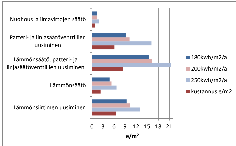
Kuva 7.7. Lämmitysjärjestelmään liittyvien korjausten ja uusimisten energiansäästö sekä toimenpiteiden hinnat 3 % energianhinnan nousulla vuodessa.
