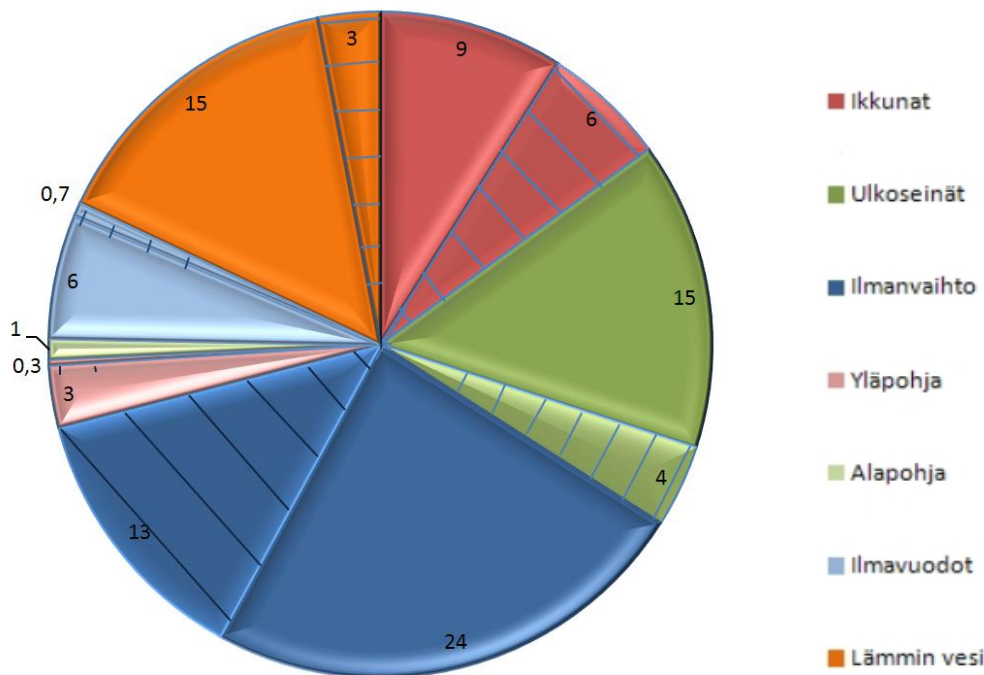
Kuva 8.3. Korjaustoimenpiteiden vaikutus tyypilliseen 1970-luvun kerrostaloon.
