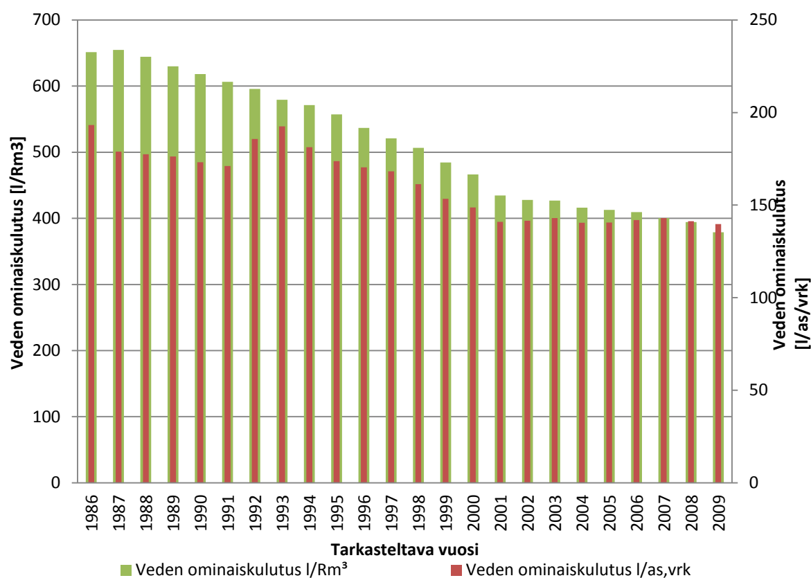
Kuva 3.7. Vedenkulutus ajanjaksona 1986-2009 (Tutkimuksen kiinteistötietokanta).
