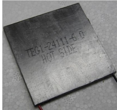
Kuva 4: Kaupallinen TEG-elementti, jonka nimellisteho on 18 W [27].
