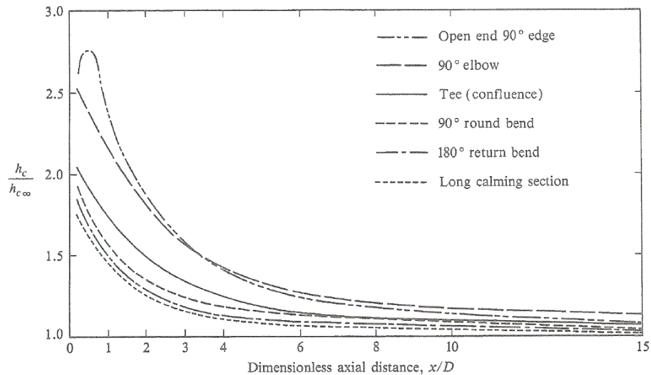
Kuva 11: Putkivirtauksen sisääntulon geometrian vaikutus lämmönsiirtokerroimeen putken alussa [36].
