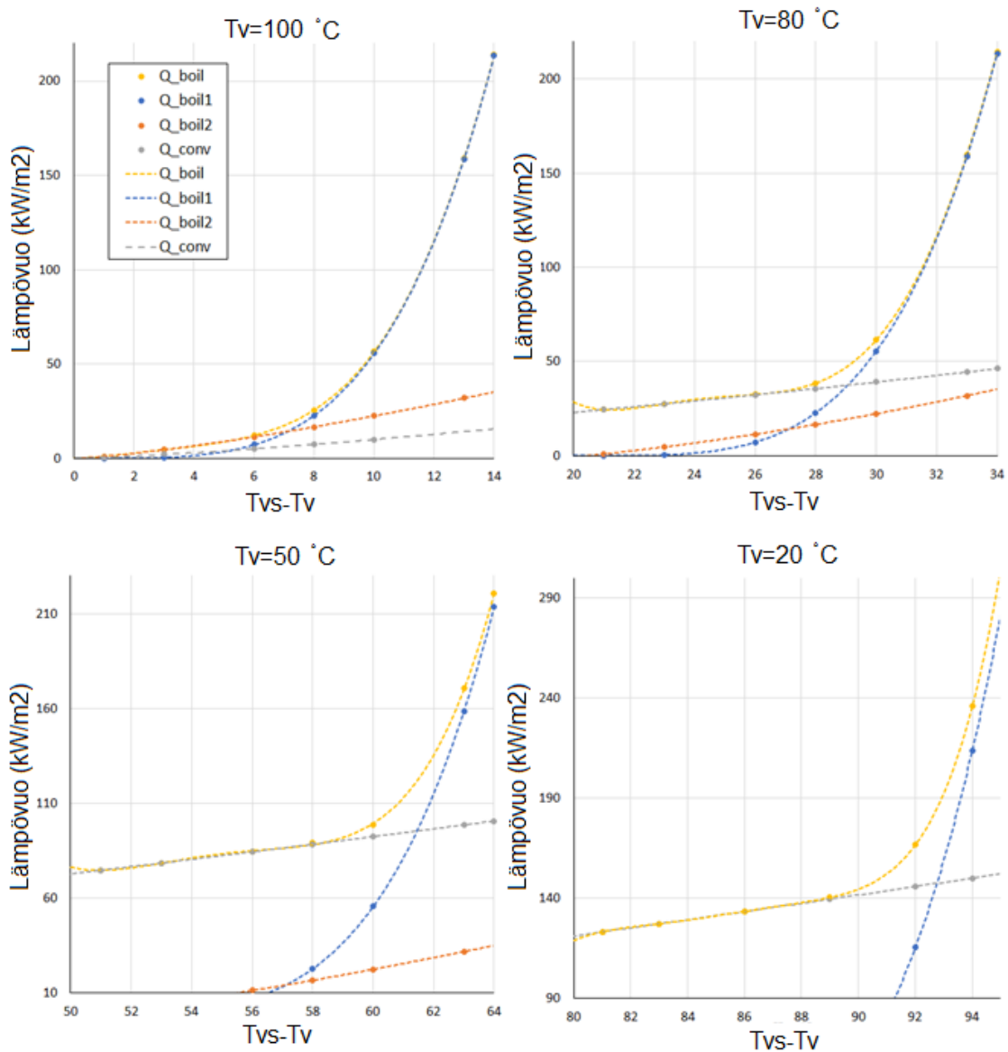
Kuva 13: Kiehumisen Q lämpötilaeron T_{vs}-T_v funktiona neljällä eri veden lämpötilalla kappaleissa 4.4.1 – 4.4.4 esitettyjen mallien mukaisesti.
