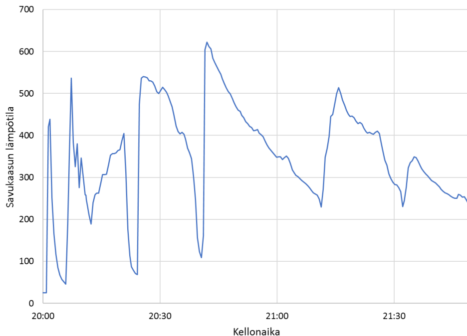
Kuva 17: Savukaasun lämpötilat 10\text{ m}^3 sisäsaunassa, kiuas tarkoitettu 8\text{-}16\text{ m}^3 tilaan. Lämpötilat mitattiin tätä työtä varten savukaasukanavasta 0,30\text{ m} etäisyydellä kiukaasta. Mittalaitteena oli Extech SD200 tallentava lämpömittari, joka oli varustettu 5\text{ mm} k-tyypin termoparianturilla.
