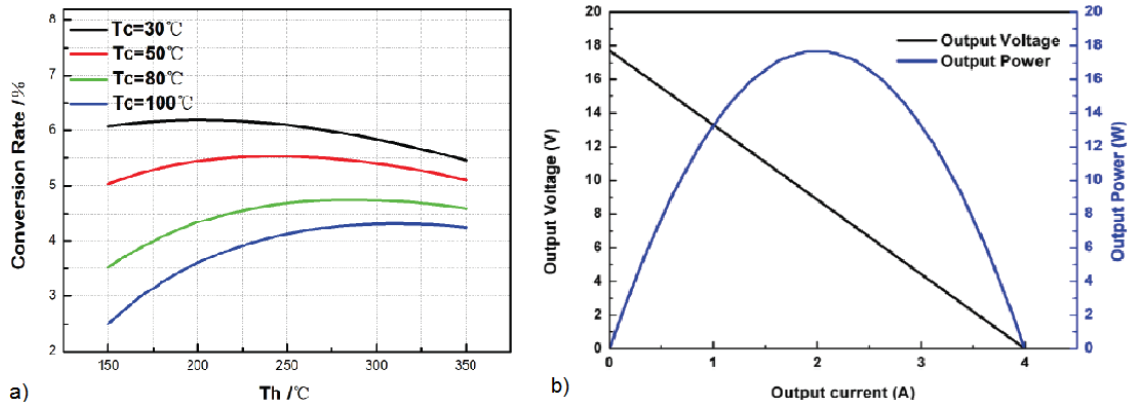
Kuva 14: a) 18 W TEG-elementin sähköntuottosuhte kuumanpuolen lämpötilan funktiona. b) Saatava teho läpi kulkevan virran funktiona, sekä tehoa vastaava ulostulon jännite-ero, kun T_h=320 ja T_c=30 . [27]
