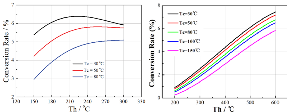
Kuva 6: BiTe- ja PbSnTe-TEG-elementtien \eta_{el} esitettyinä T_h ja T_c funktiona [32] [33].
