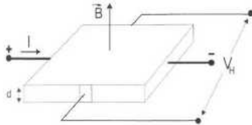
Ilustración 6 Efecto Hall. Tomado de (Moreno, 2009)
