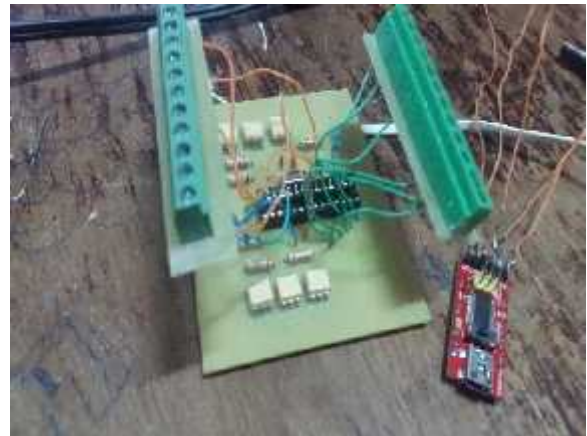
Ilustración 44 Componentes Soldados en la tarjeta
