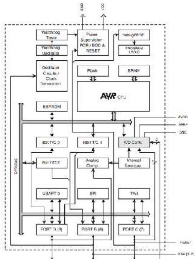
Ilustración 14 Diagrama de bloques interno Atmega 328. Tomado de http://3.bp.blogspot.com/q2TsRZDHkWO/VMpJRpRY6xl/AAAAAAAAFaw/0xzU9ZN-5uY/s1600/diagrama%2Bmicro.jpg
