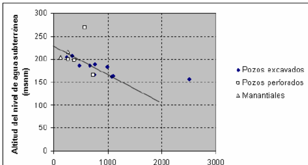
Figura 6. Relación de la altitud del nivel de agua y la conductividad eléctrica (Tomado de UNICEF, 2004).
