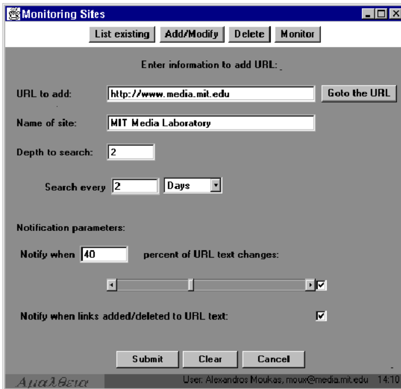
Kuva 15 Amalthea-prototyypin konfigurointikäyttöliittymä
