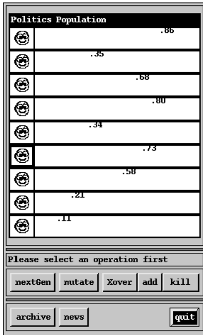
Kuva 26 NewT-ohjelman konfigurointikäyttöliittymä
