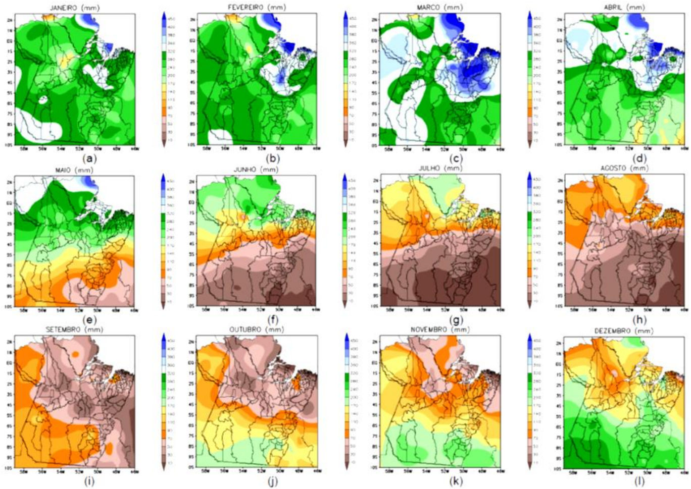
Figura 4. Padrão do regime pluviométrico mensal no Pará.
