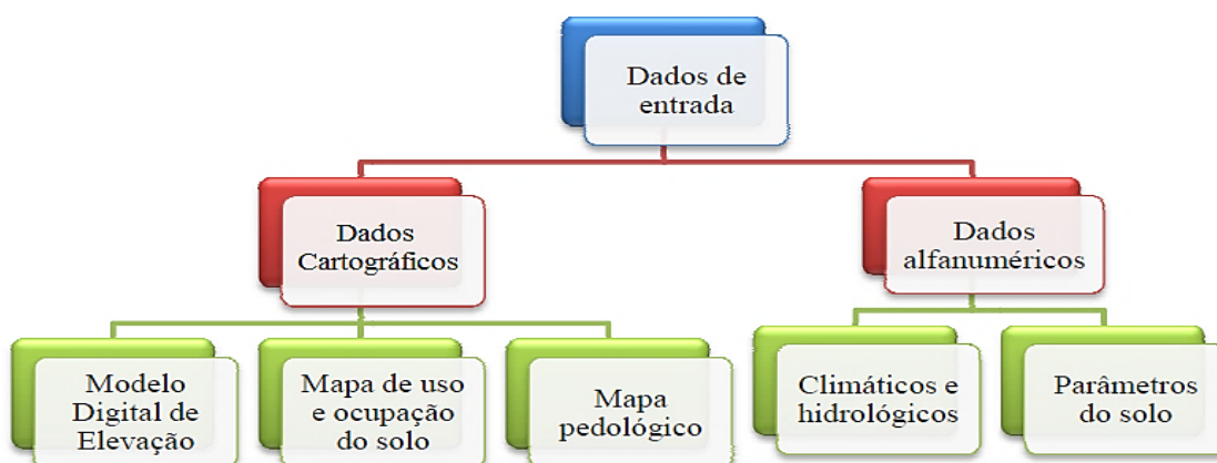
Figura 8. Fluxograma esquemática das etapas realizadas pelo SWAT.
