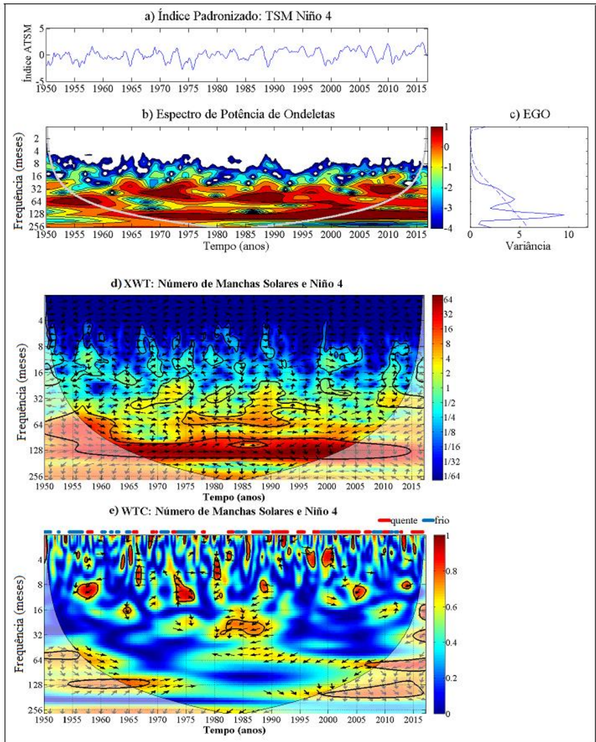
Figura 4.6: (a) Série temporal da média móvel da ATSM na região Niño 4 para o período de 1950-2016 e seu respectivo (b) Espectro de Potência de Ondeletas, menor energia (azul) e maior intensidade de energia (vermelho). (c) Espectro Global de Ondeletas (EGO), a linha pontilhada em (c) representa o intervalo de confiança do EGO (95%). (d) Transformada Ondaleta Cruzada (XWT), as cores indicam a covariabilidade de energia máxima (vermelho) e mínima (azul) entre o Número de Manchas Solares (NMS) e da ATSM na região Niño 4 e (e) Transformada Ondaleta Coerência (WTC), as cores indicam a coerência entre as duas séries que varia de 0 (azul) a 1 (vermelho). O contorno preto grosso designa o nível de significância de 5% em relação ao ruído vermelho e o Cone de Influência (COI) representado pela linha em formato de arco. As setas indicam as diferenças de fases entre as duas séries. Acima da Figura WTC, linha com a evolução no tempo dos períodos classificados como frios (azul) e quentes (vermelho) para essa região.
