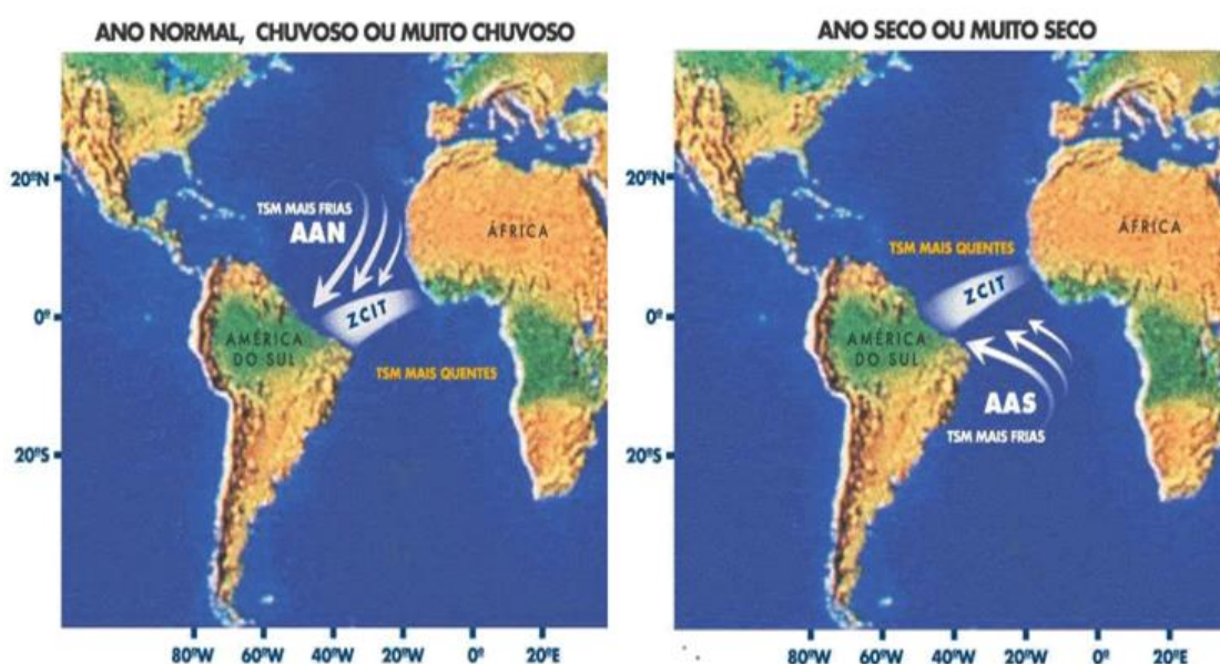
Figura 2.11: Esquema do padrão oceânico e atmosférico sobre a bacia do Oceano Atlântico.
