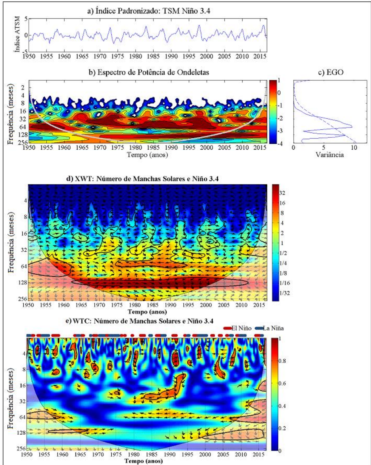
Figura 4.7: (a) Série temporal da média móvel da ATSM na região Niño 3.4 para o período de 1950-2016 e seu respectivo (b) Espectro de Potência de Ondeletras, menor energia (azul) e maior intensidade de energia (vermelho). (c) Espectro Global de Ondeletras (EGO), a linha pontilhada em (c) representa o intervalo de confiança do EGO (95%). (d) Transformada Ondaletra Cruzada (XWT), as cores indicam a covariabilidade de energia máxima (vermelho) e mínima (azul) entre o Número de Manchas Solares (NMS) e da ATSM na região Niño 3.4 e (e) Transformada Ondaletra Coerência (WTC), as cores indicam a coerência entre as duas séries que varia de 0 (azul) a 1 (vermelho). O contorno preto grosso designa o nível de significância de 5% em relação ao ruído vermelho e o Cone de Influência (COI) representado pela linha em formato de arco. As setas indicam as diferenças de fases entre as duas séries. Acima da Figura WTC, linha com a evolução no tempo dos períodos classificados como El Niño (vermelho) e La Niña (azul) pela NOAA.
