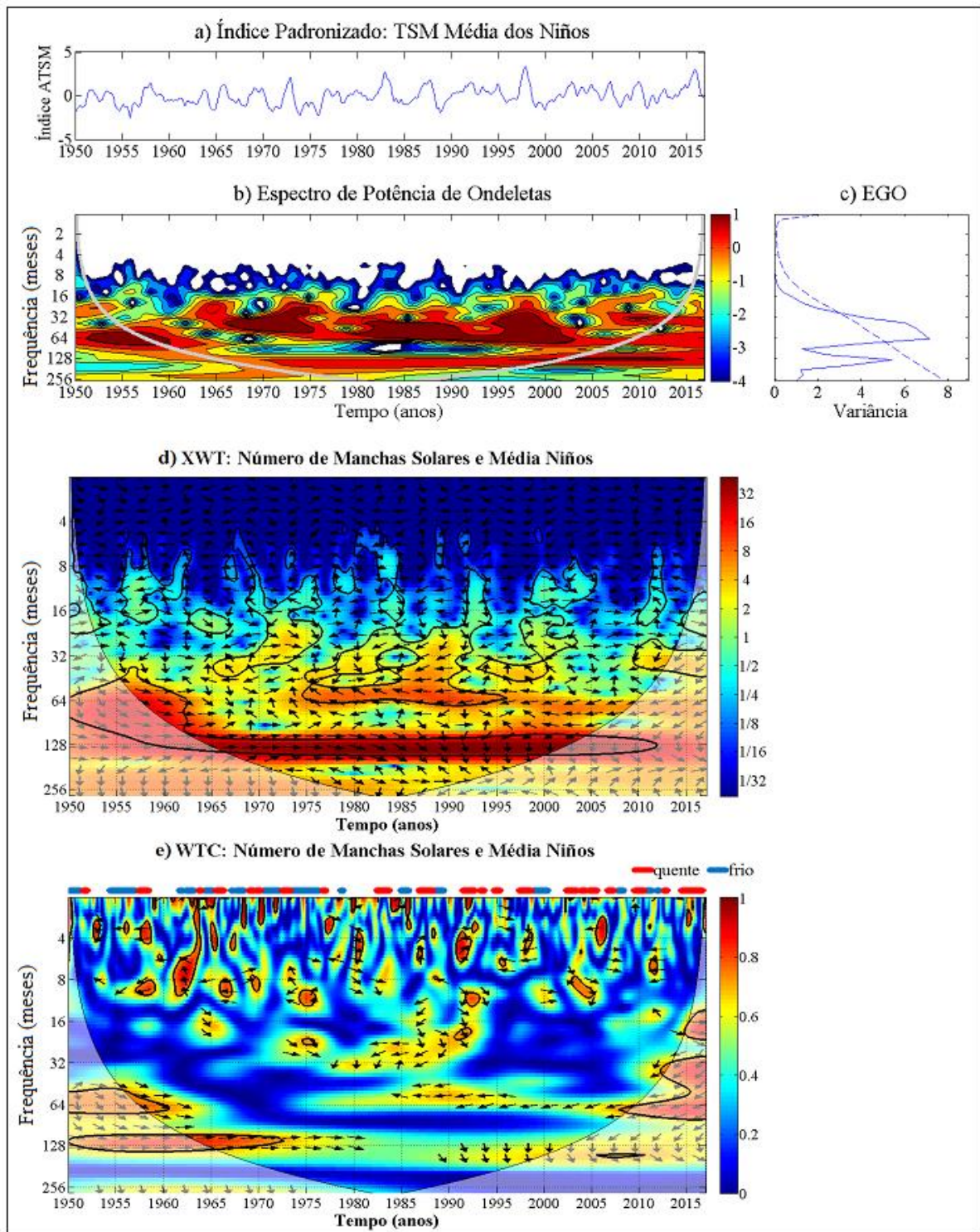
Figura 4.8: (a) Série temporal da média móvel da ATSM na região dos Niños para o período de 1950-2016 e seu respectivo (b) Espectro de Potência de Ondaletas, menor energia (azul) e maior intensidade de energia (vermelho). (c) Espectro Global de Ondaletas (EGO), a linha pontilhada em (c) representa o intervalo de confiança do EGO (95%). (d) Transformada Ondaleta Cruzada (XWT), as cores indicam a covariabilidade de energia máxima (vermelho) e mínima (azul) entre o Número de Manchas Solares (NMS) e da ATSM na região dos Niños e (e) Transformada Ondaleta Coerência (WTC), as cores indicam a coerência entre as duas séries que varia de 0 (azul) a 1 (vermelho). O contorno preto grosso designa o nível de significância de 5% em relação ao ruído vermelho e o Cone de Influência (COI) representado pela linha em formato de arco. As setas indicam as diferenças de fases entre as duas séries. Acima da Figura WTC, linha com a evolução no tempo dos períodos classificados como frios (azul) e quentes (vermelho) para essa região.
