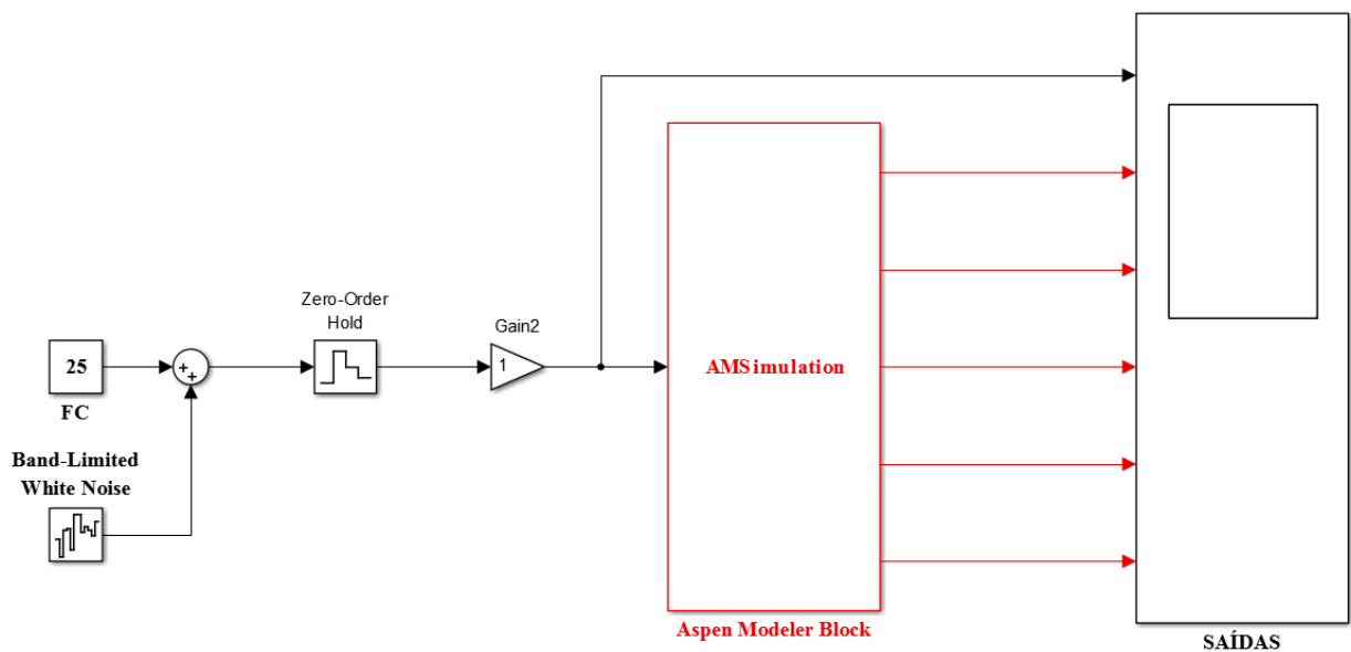
Figura 4.8 – Estrutura da comunicação Aspen-Simulink para o controle descentralizado
