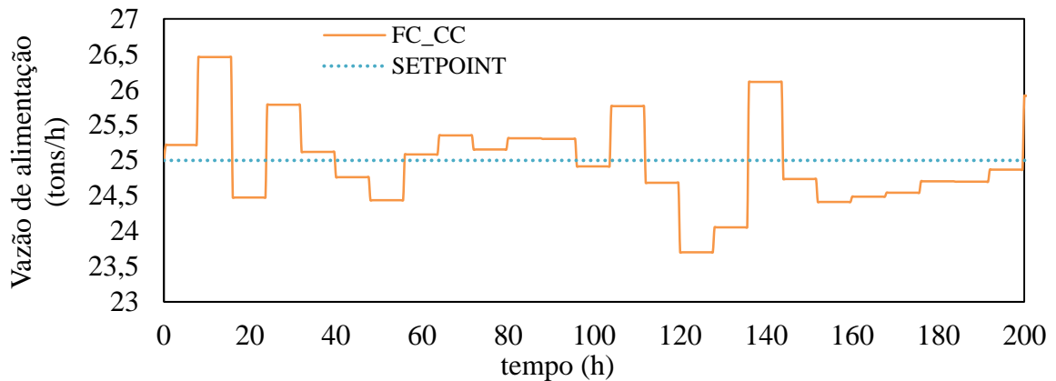
Figura 4.9 – Comportamento da vazão de alimentação (FC_CC) após o distúrbio
