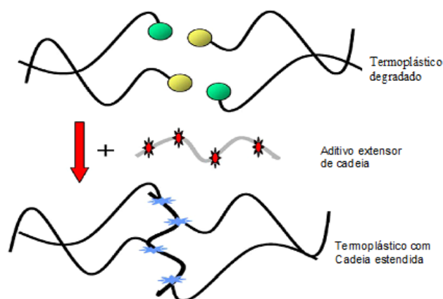
Figura 3.2 - Representação esquemática da reação de extensão de cadeia.
