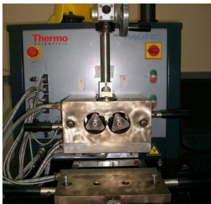
Figura 4.2 - Misturador interno acoplado ao reômetro de torque Haake Rheomix 3000QC da PolyLab QC.
