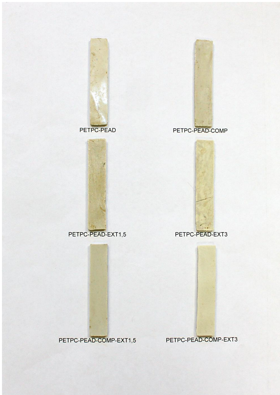
Figura 5.10 - Fotografia dos corpos de prova de impacto das misturas de PET-PC-PEAD preparadas na ausência e na presença de compatibilizante, extensor de cadeia e da combinação de compatibilizante com extensor de cadeia.
