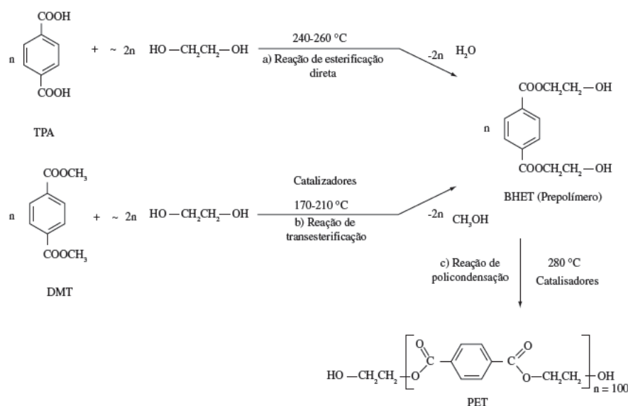
Figura 3.1 - Método de preparação do PET.
