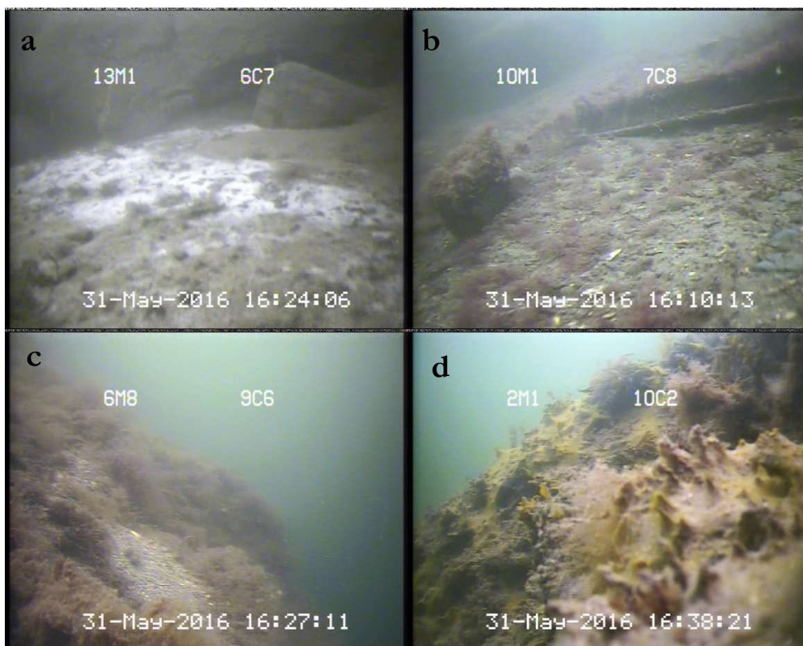
Figur 11. Skjermbilder tatt fra undervannsfilmene i område 2. a. Overgang mellom bløtbunn med hvitt bakteriebelegg, og fjellbunn med massiv nedslamming (50-90 %) b. Metallsøppel med mye nedslamming (20-50 %) og rødalger med noe nedslamming (<20 %) på skrånende sandbunn. c. Massivt nedslammet fjellbunn med algevegetasjon som er mye nedslammet. d. Fjellbunn med alger med massiv nedslamming. Det er også et grønt «teppe» med blågrønnalger som dekker algene.
