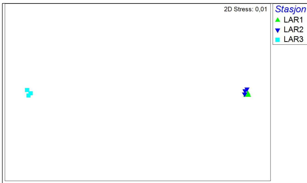
Figur 6 MDS (non-metric multi-dimensional scaling) hvor samtlige grabbprøver fra de tre stasjonene fra undersøkelsen ved Kastet i Mørjefjorden (2016) er inkludert. Plottet er basert på rot-transformerte data og Bray-Curtis likhetsmatrise, og laget med programmet PRIMER 6 (PRIMER-E, Plymouth). Plottet viser hvilke stasjoner som ligner hverandre mht. artssammensetningen. Stasjoner som ligger nærmere hverandre i MDS-plottet har likere artssammensetning enn stasjoner som ligger lenger fra hverandre.
