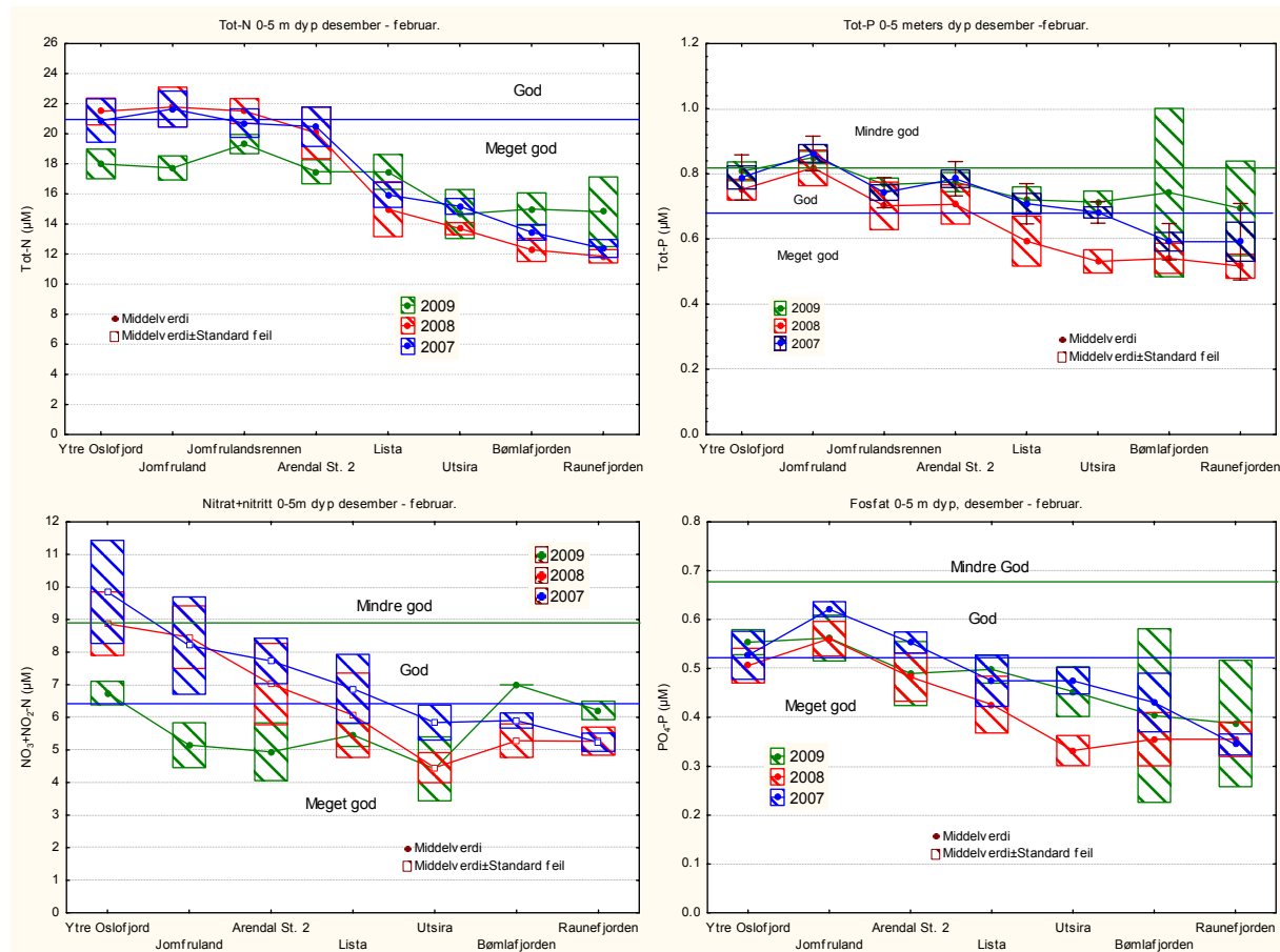
Figur 4.18. Vinterverdier av total nitrogen (Tot-N), total fosfor (Tot-P), nitrat (NO 3 +NO 2 ) og fosfat (PO 4 ) i overflatevann (0-5 m) i 2007-2009 på stasjonene Torbjørnskjær, Jomfruland, Arendal st 2, Lista, Utsira, Bømlafjorden* og Raunefjorden*. * = FerryBox-målinger (vannprøver).
