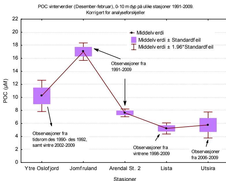
Figur 4.3. Gjennomsnittlige POC-konsentrasjoner vinterstid (0-10 m dyp) på alle stasjoner. POC-observasjonene er korrigerte for analyseforskjeller mellom laboratorier (se datarapporten for 2009).
