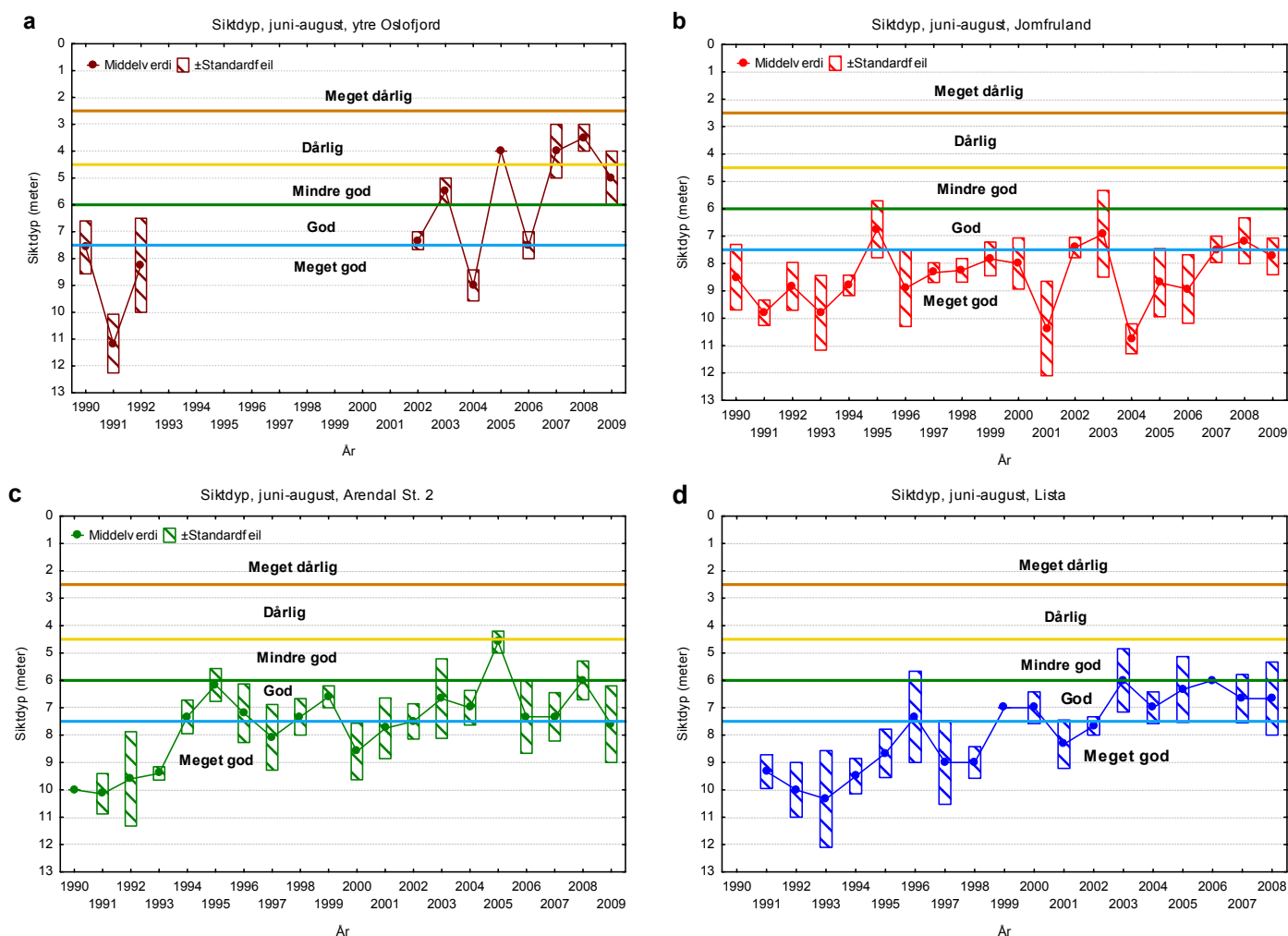
Figur 4.8 Siktdyp målt i kystvannet i Skagerrak i sommerperioden juni-august 1990-2009. a) Siktdyp ved Torbjørnskjær (Ytre Oslofjord), b) Jomfruland, c) Arendal, d) Lista. Klassifiseringen er iht. Klifs kvalitetskriterier.
