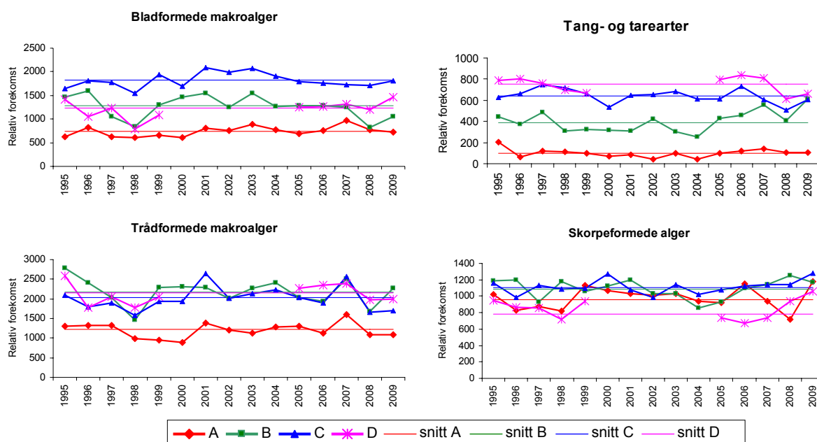
Figur 6.6. Endringer over tid i (relativ) forekomst av makroalgekategori i regionene A-D. Snittverdi er over perioden 1995-2008. (Område D er ikke undersøkt i perioden 2000-2004)
