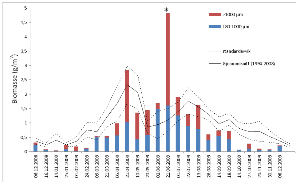
Figur 5.14. Dyreplanktonbiomasse som tørrvekt ( \text{g/m}^2 ) for de øvre 50 m Fordelt på to størrelsesfraksjoner, 180- 1000 \mu\text{m} og 1000 \mu\text{m} , i 2009 på Arendal St.2. * Relativt høy verdi for >1000 \mu\text{m} fraksjonen 21.06 er sannsynligvis forårsaket av høy algebiomasse i prøven. Gjennomsnitt og standardavvik er vist for perioden 1994-2008.
