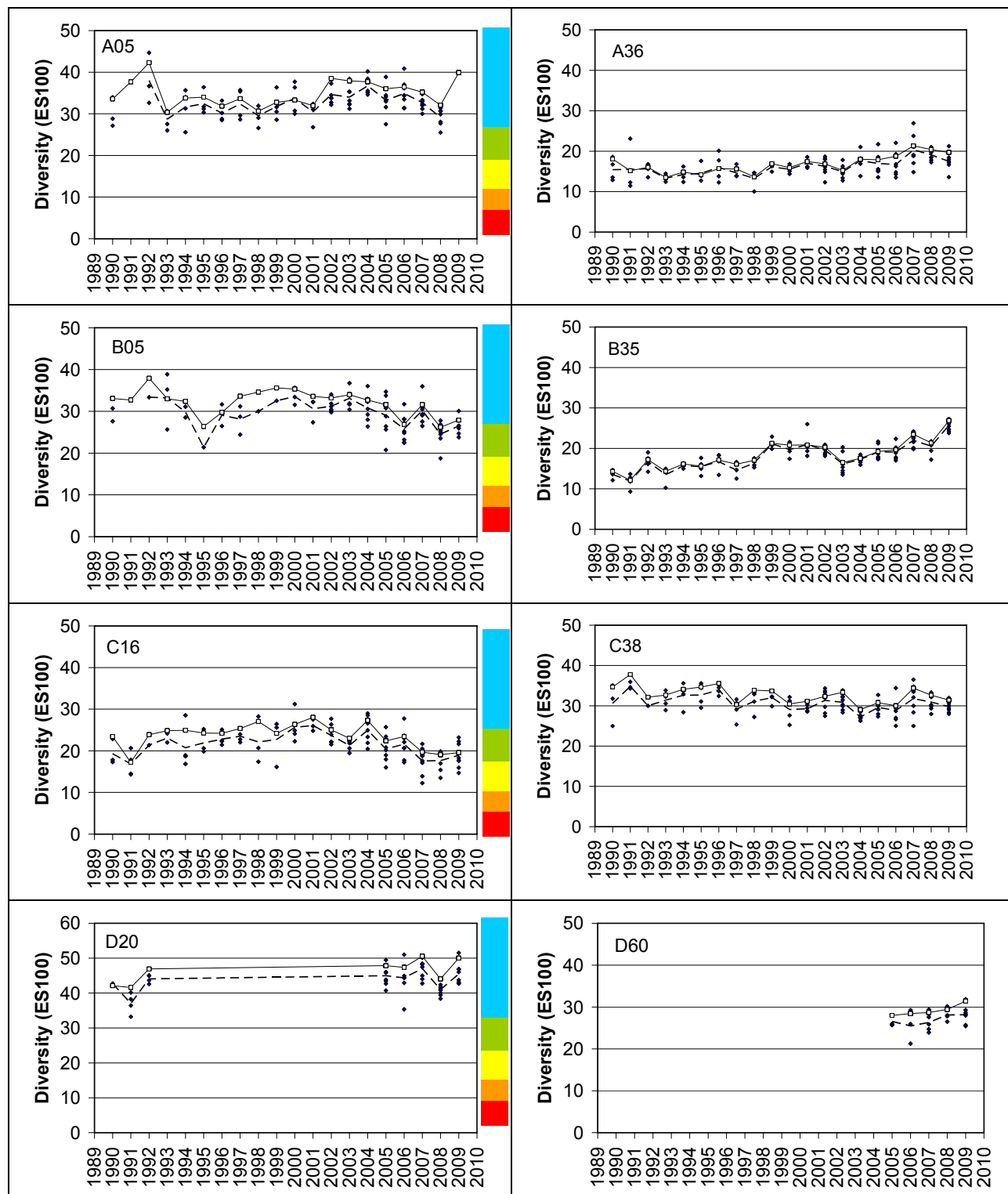
Figur 7.3. Hurlberts diversitetsindeks (artstall pr. 100 individer, ES_{100} ) 1990-2009. Punkter: Verdier pr. grabb. Prirkete linjer: Gjennomsnitt for parallelle grabber. Heltrukket linje og åpne punkter: Verdier for stasjonen (sammenslåtte grabber). Fargene angir tilstandsklasser (se Figur 7.2). Merk at verdier pr. grabb ikke kunne beregnes på stasjon A05 i 2009 fordi prøvene hadde <100 individer.
