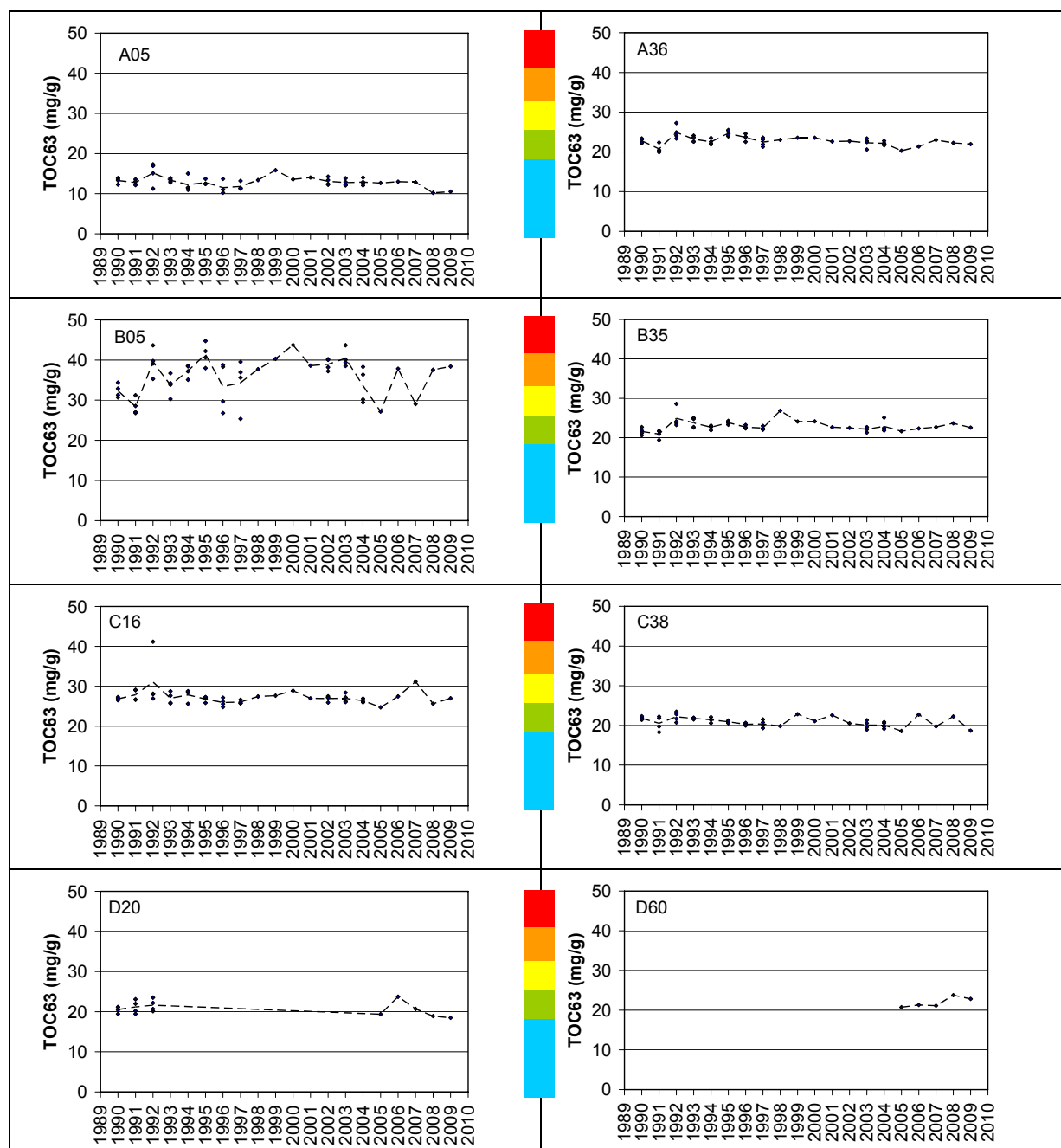
Figur 7.11. Innhold av totalt organisk karbon (TOC 63 , mg/g), korrigert for sedimentets innhold av silt og leire i enkeltprøver (punkter) og som gjennomsnitt (linjer) pr. år 1990-2009 (som følge av nye retningslinjer for prøvetaking er prøvene i 2009 tatt fra 0-5 cm for kornstørrelse og 0-1 cm for TOC, mens både kornstørrelse og TOC tidligere ble tatt fra 0-2 cm). På B-stasjonene er både TOC og kornstørrelse tatt fra 0-5 cm i 2009). Fargekodene angir tilstandsklasser (se Figur 7.2).
