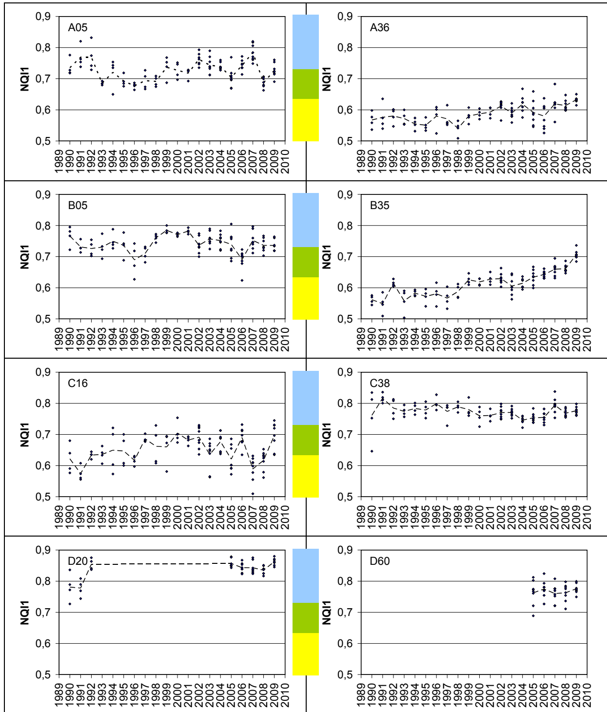
Figur 7.10. Norsk kvalitetsindeks (NQI1) for bløtbunnsfauna pr. grabb 990-2009. Punkter: Verdier pr. grabb. Prikkede linjer: Gjennomsnitt for parallelle grabber. Fargene angir tilstandsklasser (se Figur 7.2, Klassifisering iflg. Molvær et al. 2008.)
