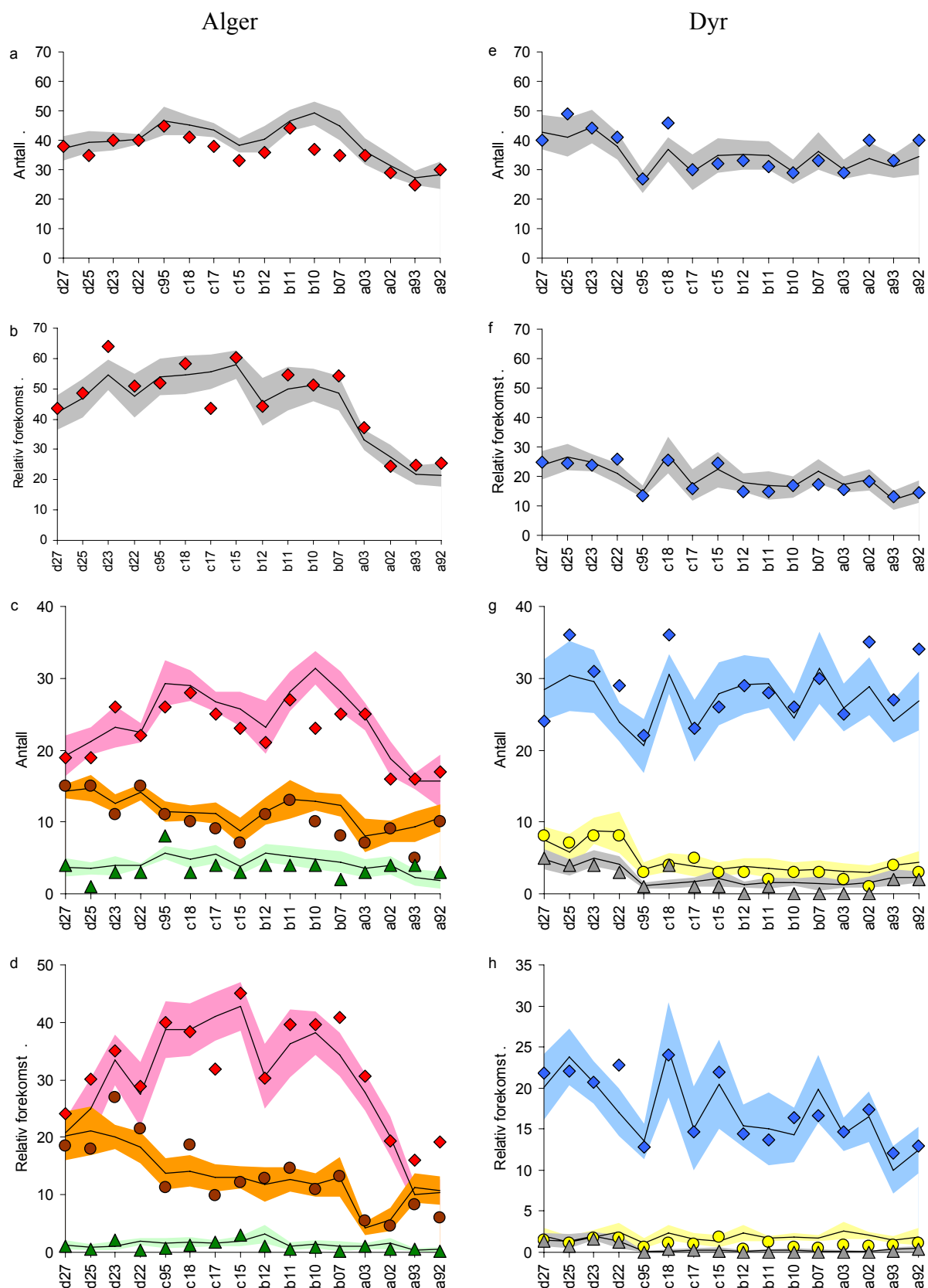
Figur 6.2. Antall arter og forekomst av makroalger og dyr i 2009 i dybdeintervallet 4-22 m. Punkter = 2009-observasjoner. Linje m/farget felt = gjennomsnitt og standardavvik (1995-2008). a) antall arter og b) forekomst alger, c) antall arter og d) forekomst av rødalger (rød), brunalger (brun) og grønnalger (grønn), e) antall arter og f) forekomst dyr, g) antall arter og h) forekomst av vannfiltrerere (blå), rovdyr/altetende (gul) og beitere (grå).
