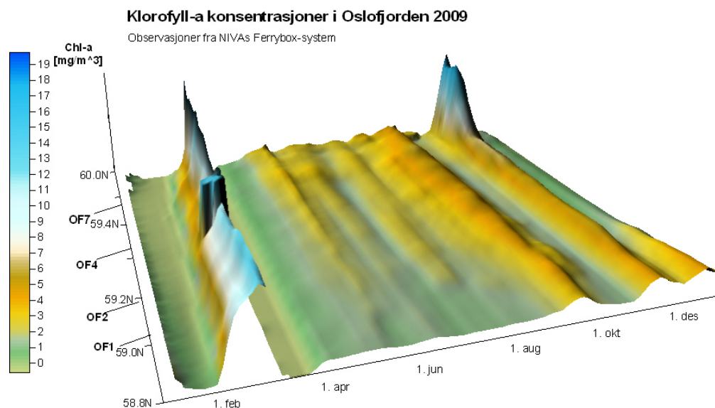
Figur 5.1. Klorofyll-a i Ytre Oslofjord fra Breidangen (OF7) til Torbjørnskjær (OF1) basert på Ferrybox klorofyll-a fluorescence data fra Color Fantasy. Posisjoner til faste stasjoner fra Filtvedt (OF7) til Torbjørnskjær (OF1) er markert.
