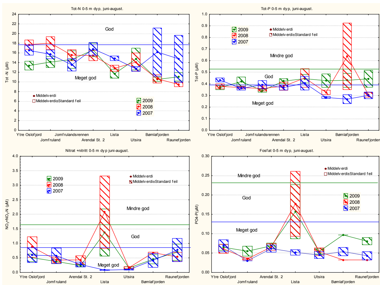
Figur 4.19. Sommerverdier av total nitrogen (Tot-N), total fosfor (Tot-P), nitrat ( \text{NO}_3+\text{NO}_2 ) og fosfat ( \text{PO}_4 ) i overflatevann (0-5 m) i 2007-2009 på stasjonene Torbjørnskjær, Jomfruland, Arendal st 2, Lista, Utsira, Bømlafjorden* og Raunefjorden*. * = FerryBox-målinger.
