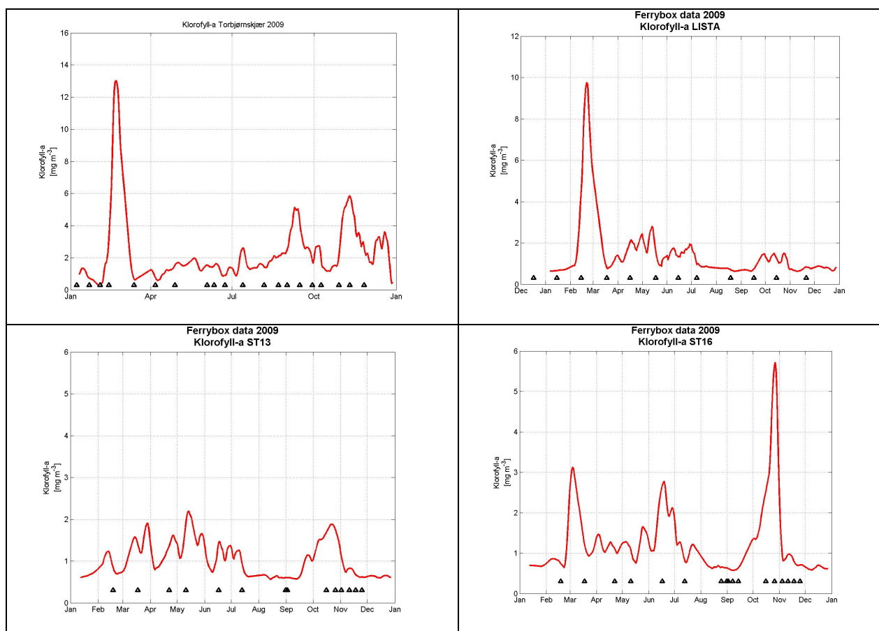
Figur 5.2. Klorofyll-a ( \mu\text{g/l} ) ved Torbjørnskjær (Ytre Oslofjord), Lista, Bømlafjorden (St. 13) og Raunefjorden (St.16) i 2009. De røde linjene illustrerer Ferrybox-observasjoner (7 dagers glidende middel av døgnmedian). Tidspunkt for manuell eller hydrografisk prøvetaking er markert.
