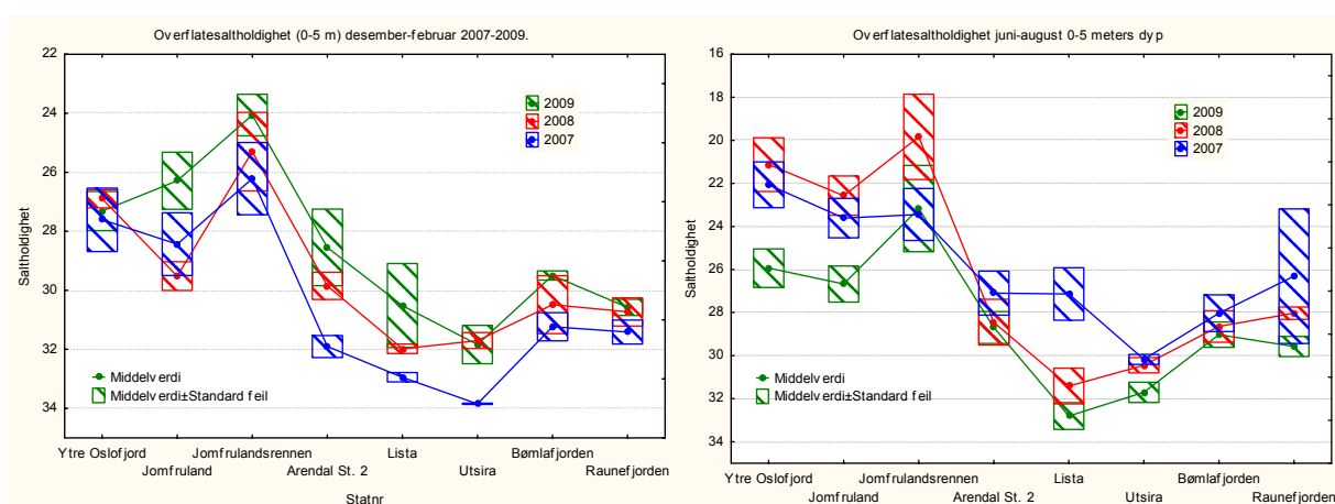
Figur 4.16. Saltholdighet i overflatevann (0-5 m) vinter (venstre figur) og sommer (høyre figur) 2007, 2008 og 2009.
