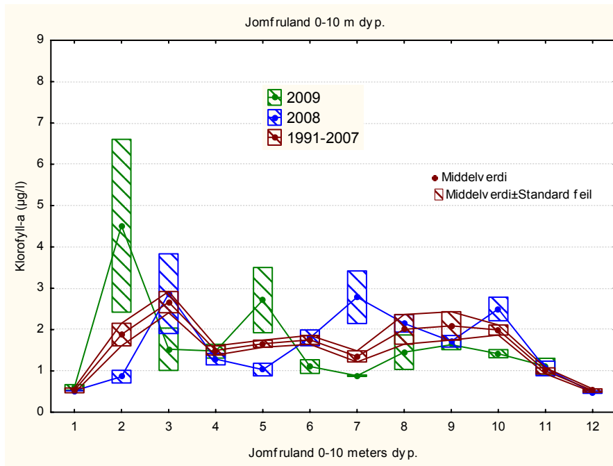
Figur 4.21b Månedlig planteplanktonbio- masse (klorofyll-a) i overflatevann (0- 10 m) på stasjon Jomfruland i 2008 og 2009 sammenliknet med perioden 1991- 2007.
