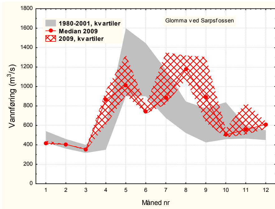
Figur 3.8 Månedsvannføring i Glomma i 2009 sammenlignet med gjennomsnittlig vannføring fra 1980-2001 (Data fra NVE og Glommens og Laagens Bruks-eierforening (GLB)).
