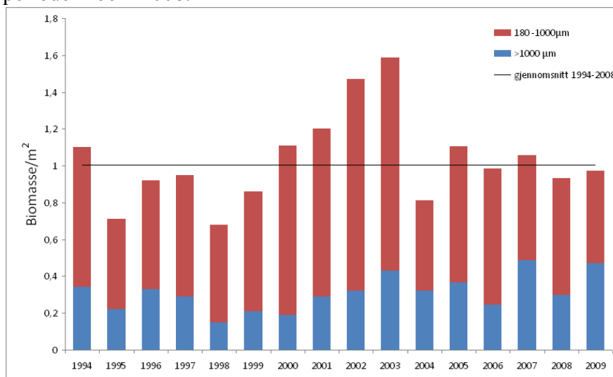
Figur 5.15 Årlig gjennomsnittlig dyreplankton biomasse ( \text{g tørrvekt/m}^2 ) for de øvre 50 m fordelt på to størrelsesfraksjoner, 180- 1000 \mu\text{m} og > 1000 \mu\text{m} , 1994-2009 på Arendal St.2. Horisontal linje viser gjennomsnitt for perioden 1994-2008.
