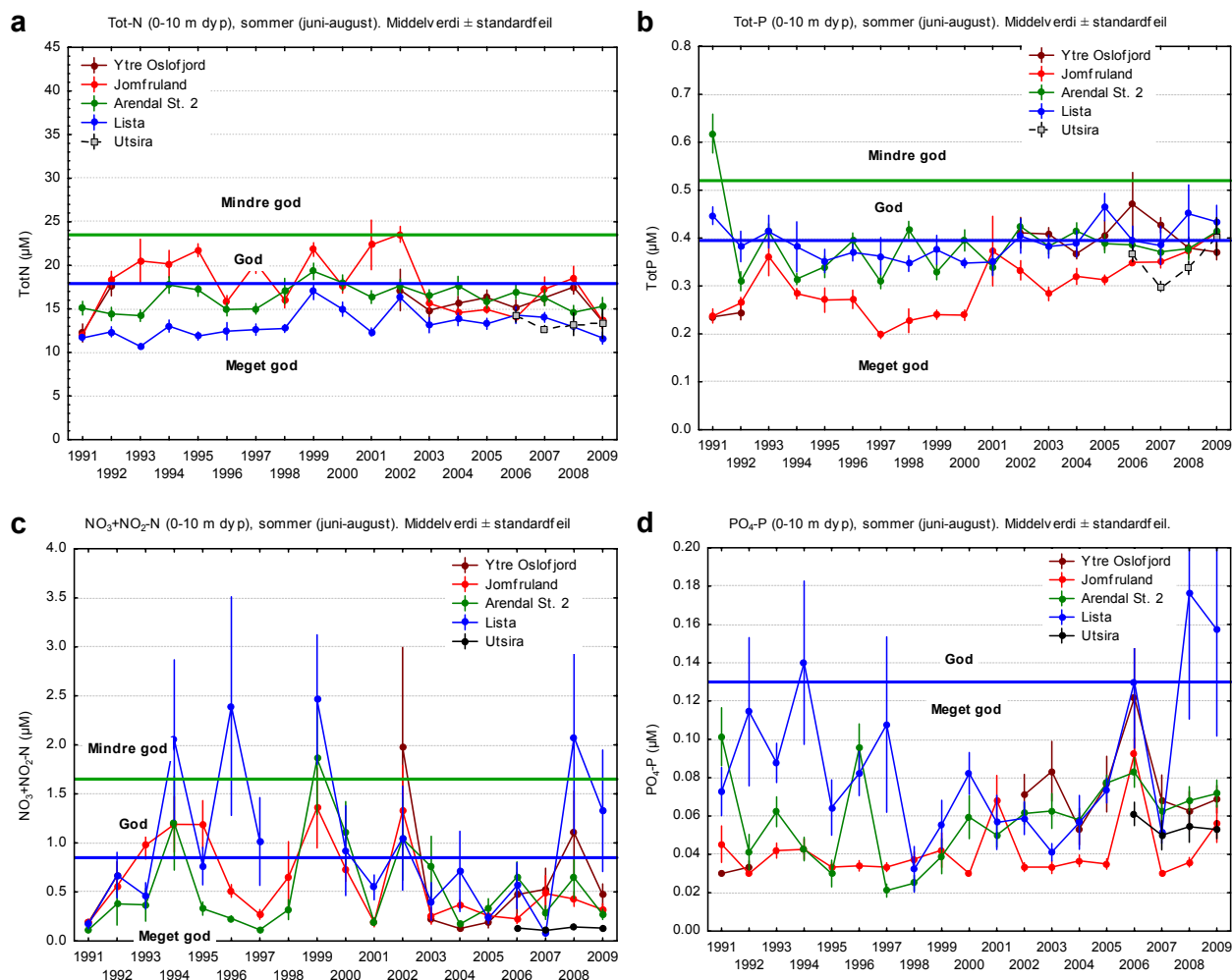
Figur 4.6. Næringsalter i overflatevann (0-10m dyp) sommerstid (juni-august) i 1991-2009. a) Tot-N, b) Tot-P, c) NO 3 +NO 2 -N og d) PO 4 -P (µM). Klifis klassifiseringsgrenser er markert.
