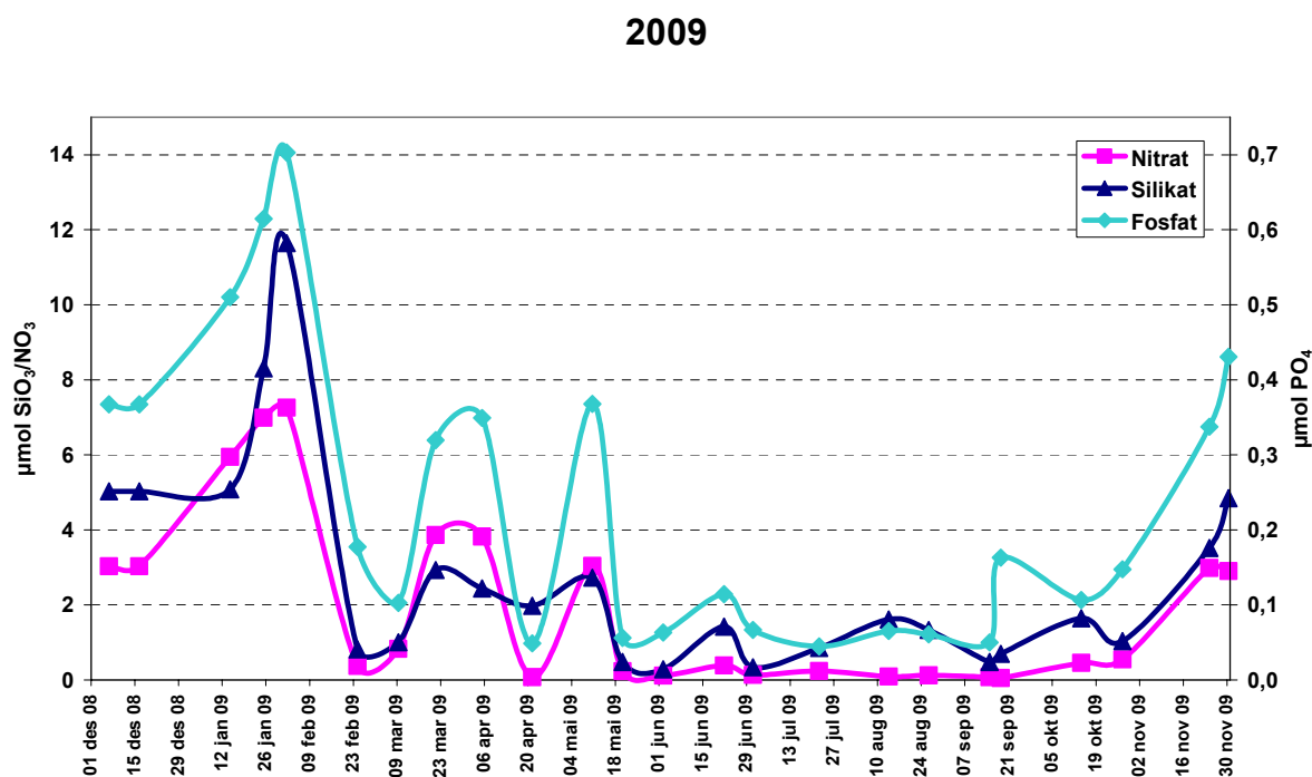
Figur 5.5. Tidsutviklingen for nærings saltene silikat, nitrat og fosfat på 5 meters dyp ved Arendal (st.2) gjennom året 2009.
