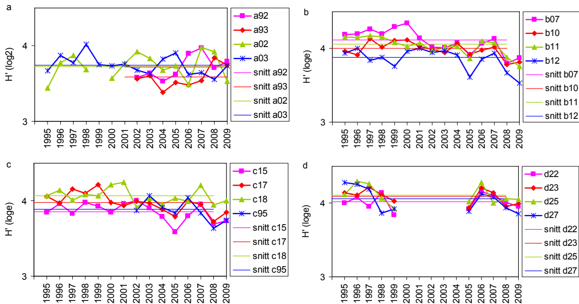
Figur 6.1. Biologisk mangfold i hardbunnssamfunn på grunt vann langs kysten av Sør-Norge i region A, B, C og D. Biomangfold er basert på Shannon-Wiener indeks H' (log 2 ) (Shannon & Weaver, 1963) og forekomst av alger og dyr er gitt som sum over dyppet av e^x hvor x er: 1=enkeltpunkt, 2=sjelden, 3=vanlig, 4=dominerende. Gjennomsnitt er beregnet for perioden 1995-2008.
