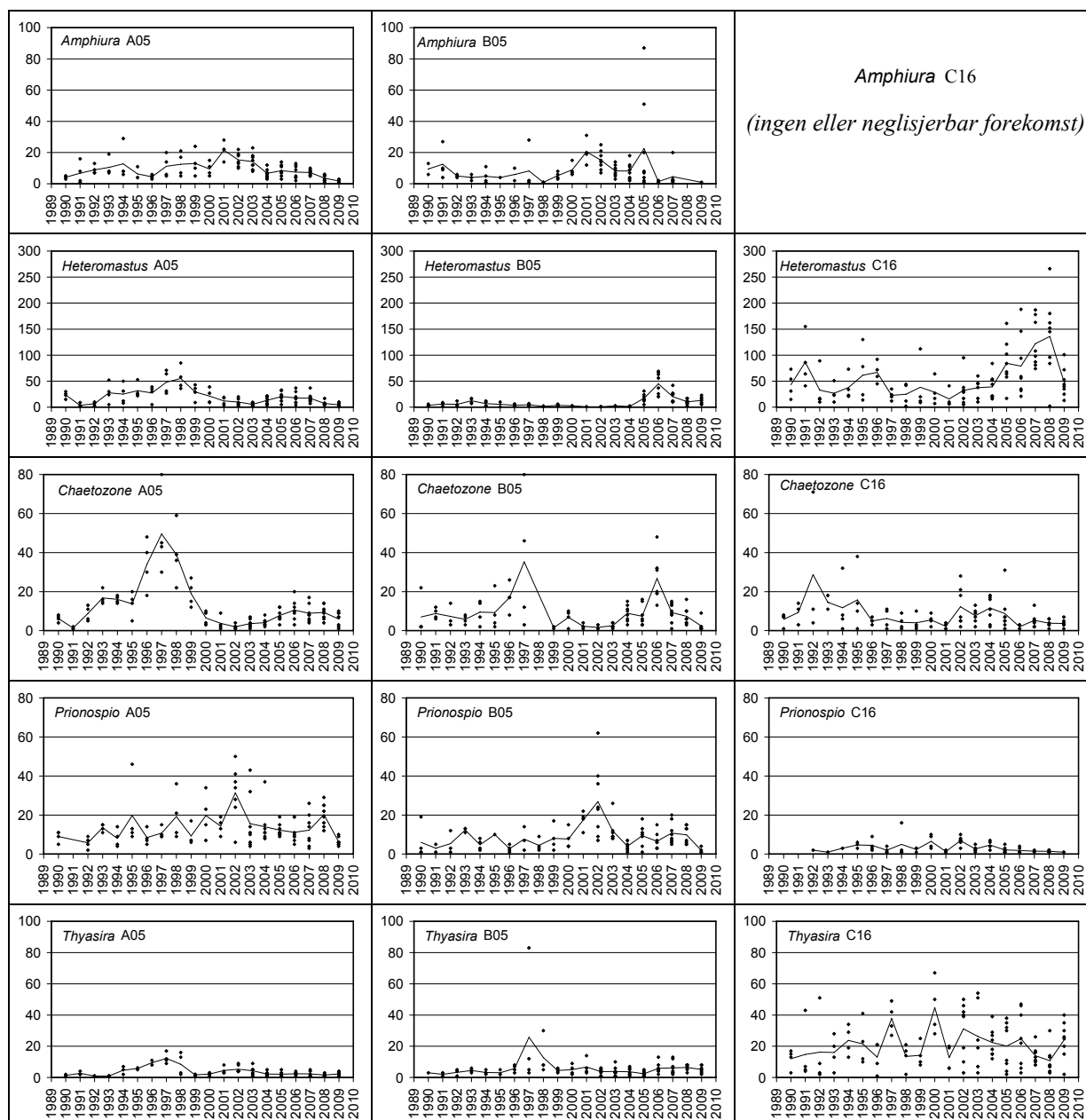
Figur 7.6. Antall individer pr. grabb (punkter) og gjennomsnitt (linje) for noen vanlige slekter på de grunne stasjonene A05 (Ytre Oslofjord, 50m), B05 (Arendal, 50m) og den middels dype fjordstasjonen C16 (Grønsfjord ved Farsund, 160m). Merk ulik skala for forskjellige slekter.
