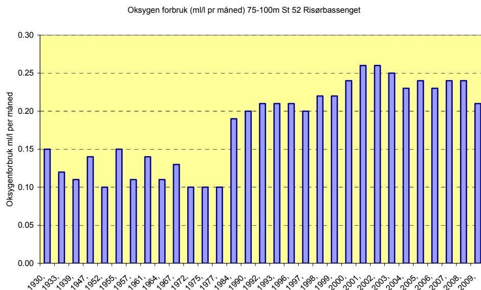
Figur 4.13. Oksygenforbruket i Risørbassenget fra 1930 til 2009 (Kilde: HI).
