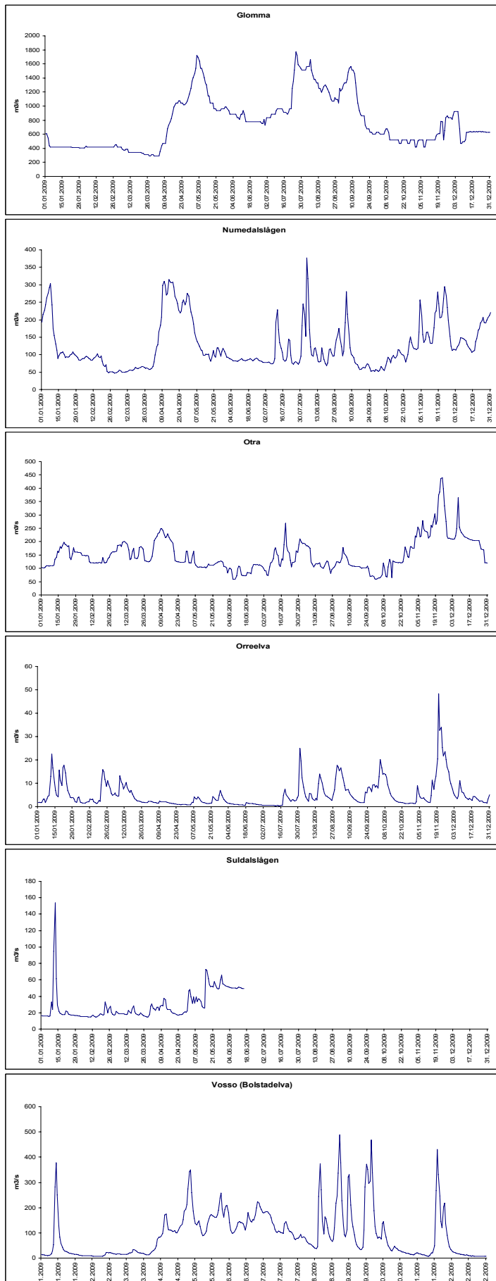
Figur 3.9. Vannføring (døgnmiddel \text{m}^3/\text{s} for 2009) i elvene Glomma, Numedalslågen, Otra, Orreelva, Suldalslågen og Vosso. Data juli-desember mangler fra Suldalslågen (Kilde: NVE).
