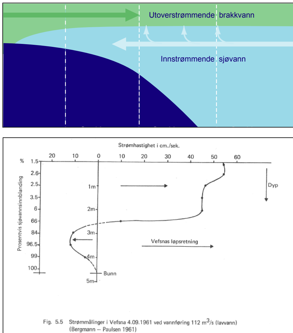
Figur 6. Beskrivelse av det to-lags strømsystemet som dannes av utstrømming av ellevann (estuarin sirkulasjon). Øvre figur: prinsippskisse. Nedre figur: Strømmålinger i Vefsnas munning 4.9.1961 ved vannføring 112 m 3 /s og lavvann (fra Bergmann-Paulsen, 1961)
