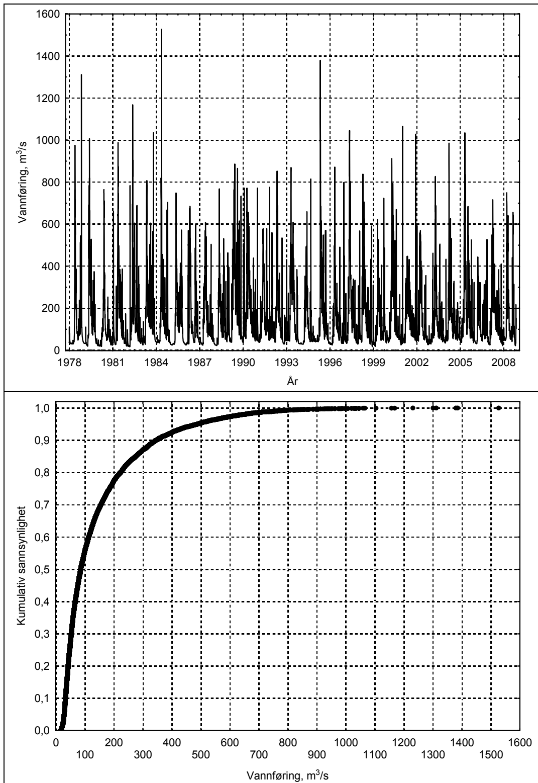
Figur 3. Vefsna vannføring med Laksfors i tidsrommet 1978-2008. Øvre figur: døgnverdier. Nedre figur: kumulativt diagram. Verdien 0,5 på y-aksen tilsvarer medianen og 0,9 tilsvarer 90-persentilen.
