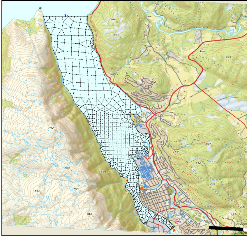
Figur B1 Nettverket eller gridet i RMA2-modellen for simulering av sirkulasjon. Nettverket består av trekanter og firkanter. I ytre del er sidelengden 20 m og i indre del er sidelengden 10 m. I hvert hjørne og midt på hver side (noder) beregnes høyden over referansedypet, strømretningen og strømhastigheten.
