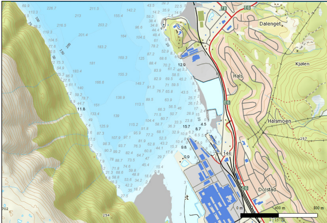
Figur 2. Dypdeforhold i Vefsnas munningsområde og i havneområdet.
