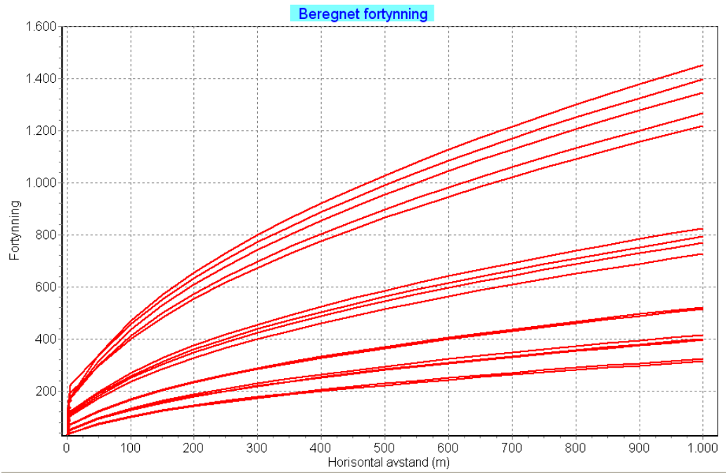
Figur 16. Beregnet fortynning av avløpsvannet ved utlipp av 33 \text{ m}^3/\text{h} og svak strøm ( 2 \text{ cm/s} )
