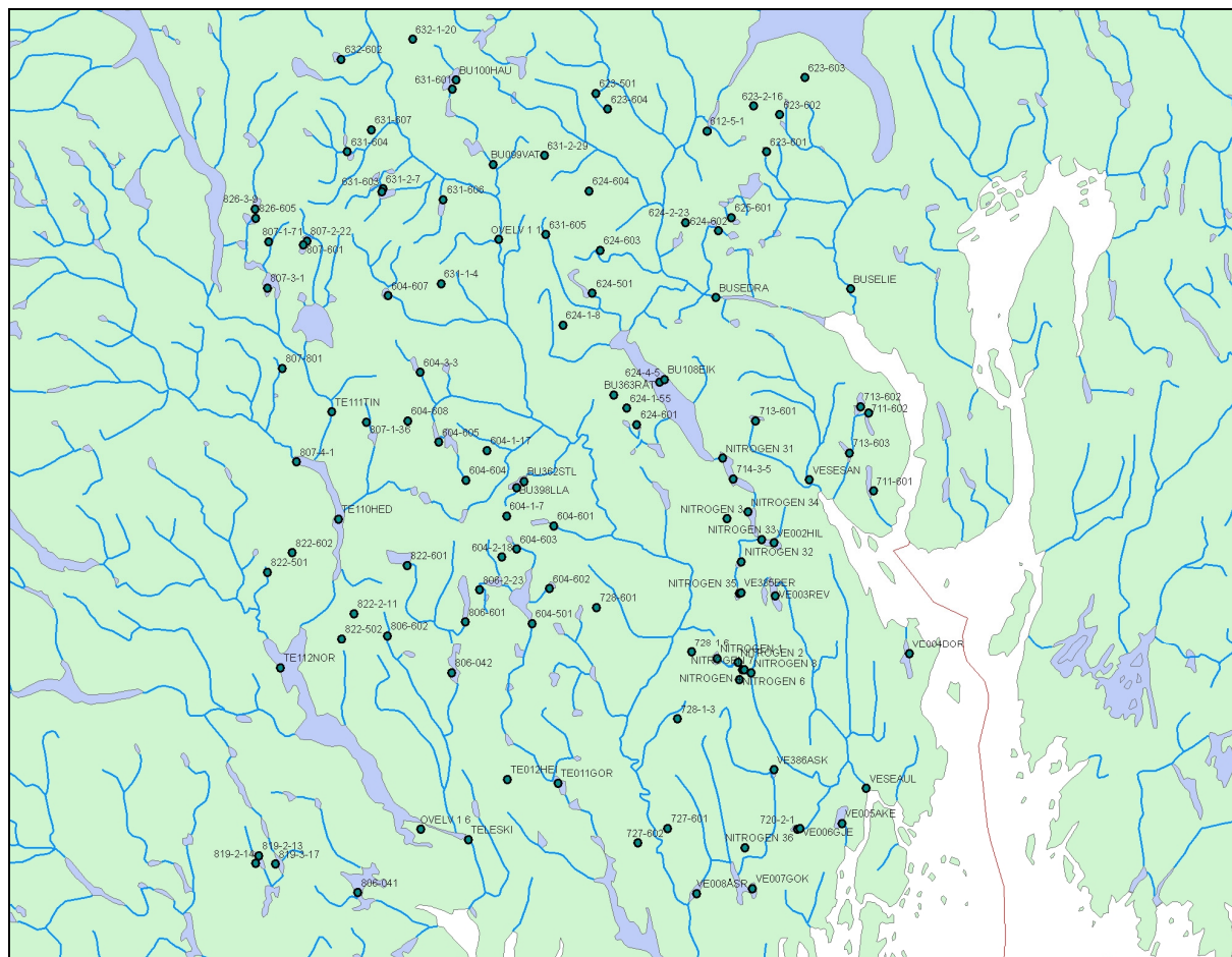
Figur 3. Utsnitt med lokaliteter der det er registrert vannkjemiske data i NIVAs RESA overvåkningsdatabase. De fleste har både Ca og TOC i tillegg til næringssalter og metaller.
