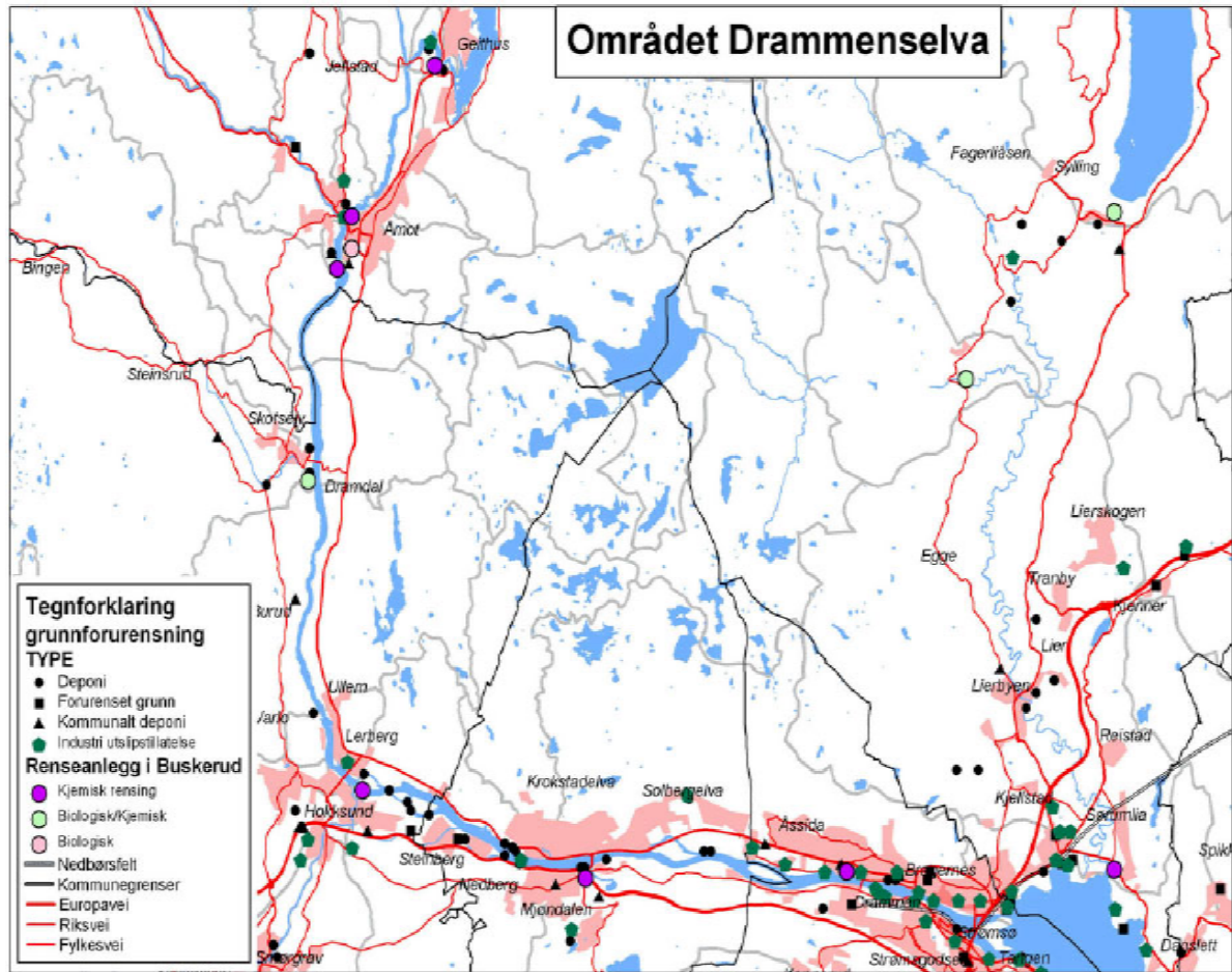
Figur 5. Kjente steder med grunnforurensning og kloakkrenseanlegg ved Drammenselva (kilde: Drammen kommune sin internettside).
