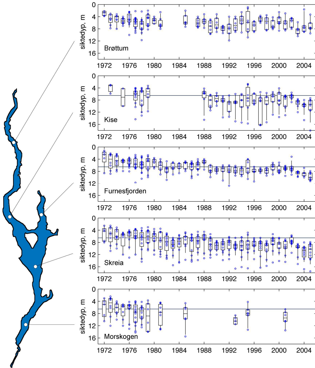
Figur 3. Tidstrend for siktedyp ved fem lokaliteter i Mjøsa i tidsperioden 1972-2005. Streken angir fastsatt nasjonalt og interkommunalt miljøkvalitetsmål for Mjøsa dvs. at siktedypet i Mjøsas midtre (Kise, Furnesfjorden og Skreia) og søndre del (Morskogen) under normale forhold ikke bør være mindre enn 6-7 meter. Vi må også nevne at nåværende interkommunale miljøkvalitetsmål for siktedypet i Mjøsas sentrale hovedvannmasser skal være > 8 meter. Dvs. at siktedypet ved stasjon Skreia (hovedstasjonen) bør være større enn 8 meter under normale forhold. Boksene viser intervallet mellom 25 og 75-prosentilene. Den horisontale streken inne i boksen viser median (50-prosentilen), mens de vertikale strekene viser intervallet mellom 10 og 90-prosentilen. I Mjøsas nordre del varierer siktedypet mye pga. naturgitte forhold og det er derfor lite hensiktsmessig å fastsette noe konkret miljøkvalitetsmål for siktedypet i denne del av innsjøen. Det største siktedyp som blitt registrert i Mjøsa i den tid ”Mjøsundersøkelsene” har pågått er på 18,0 meter som ble målt ved st. Kise den 19/5 2005. Vi kan videre nevne at klart vann og stor siktbarhet er en viktig faktor for at Mjøsa skal være et godt leveområde for storørret og godt egnet som råvann til drikkevannsproduksjon.
