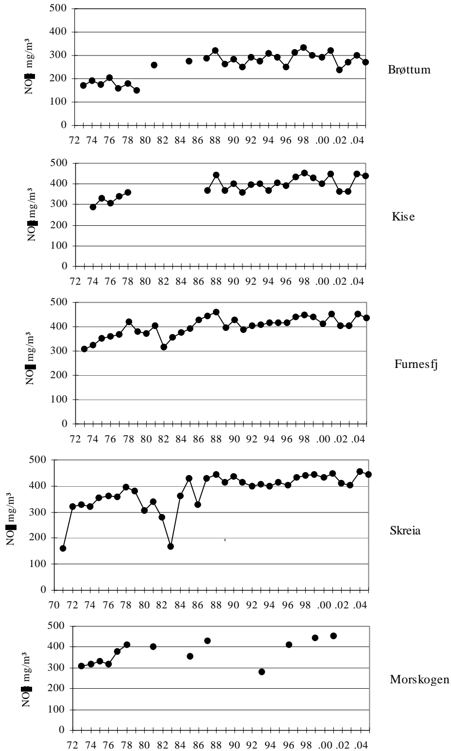
Figur 11. Middeler verdier (fra en vertikalserie fra overflaten til bunn) for nitrat fra observasjoner på senvinteren ved hovedstasjonen (Skreia) og fire supplementstasjoner (Brøttum, Kise, Furnesfjorden og Morskogen) i tidsperioden 1971-2005.
