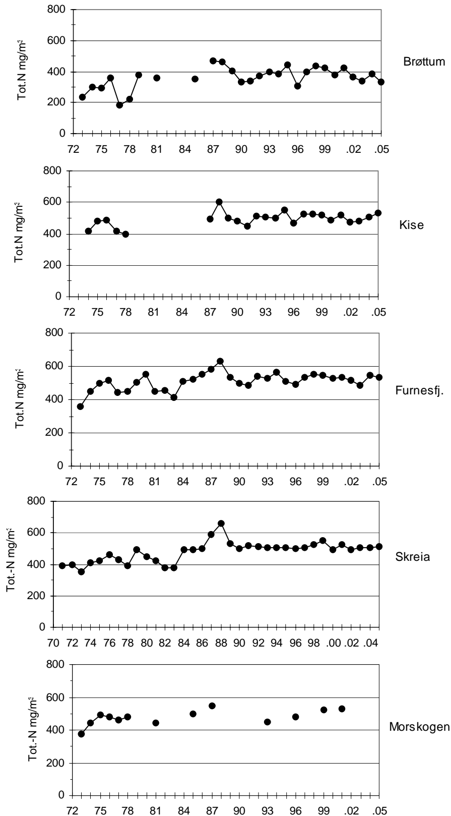
Figur 10. Middelerverdi (fra en vertikalserie fra overflaten til bunn) for total nitrogen fra observasjoner på senvinteren ved hovedstasjonen (Skreia) og fire supplementstasjoner (Brøttum, Kise, Furnesfjorden og Morskogen) i tidsperioden 1971-2005. Vurdert ut fra SFTs klassifisering av miljøkvalitet i ferskvann kan tilstanden for nitrogen i Mjøsa nå betegnes som "Mindre god". Viktigste årsak til den høye konsentrasjonen er lekkasje fra dyrket mark.
