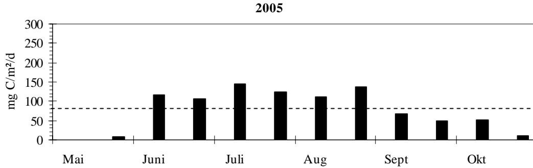
Figur 21. Primærproduksjon (beregnet ut fra C_{14} -metodik) uttrykt som døgnsproduksjon i Mjøsas sentrale del (st. Skreia) i 2005. Årsproduksjon er beregnet til 15 gram C/m^2 , maksimal døgnsproduksjon til 145 mg C/m^2 og midlere døgnsproduksjon (stiplet linje) til 81mg C/m^2 . Faglig sett, vurdert ut fra foreliggende kunnskap om Mjøsa, bør ikke den maksimale døgnsproduksjon overstige 300 mg C/m^2 , dvs. at forholdene i 2005 stort sett var i samsvar med ønsket miljøkvalitetsmål. Generelt sett så er det likevel ønskelig med så stor primærproduksjon som mulig i de frie vannmasser innenfor gitte miljøkvalitetsmål dvs. mål for algebiodiversitet og algetetthet (biomasse).
