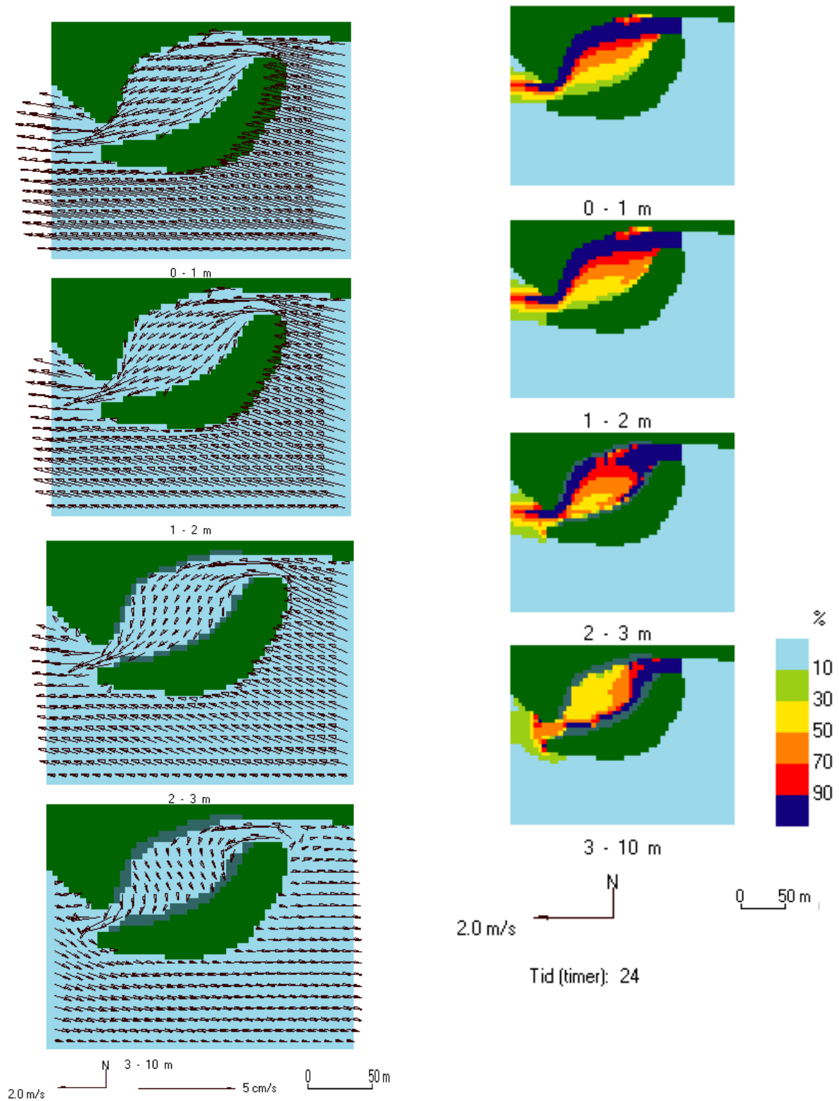
Figur 8. Vind mot vest på 2 m/s. Vannutsiftning etter ett døgn. Vannet strømmet inn gjennom åpningen i øst. God vannutveksling i hele bassenget. Best nær østlig åpning og i nordlige deler.
