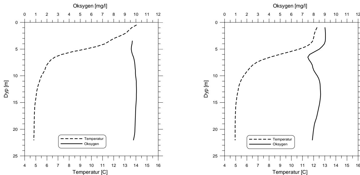
Figur 9. Temperatur- og oksygenkurver for Grasdalsvatn målt i 2000. Til venstre 22. juni; til høyre 20. september. Målingene er utført med en Seabird SBE19 sonde, og oksygenmålinger er kalibrert mot punktmålinger vha. Winklers metode.
