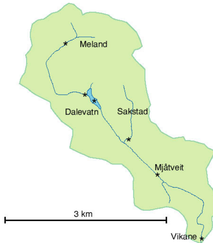
Figur 30. Mjåtveitvassdraget. Nedbørfelt og prøvestasjoner (markert med stjerne).
