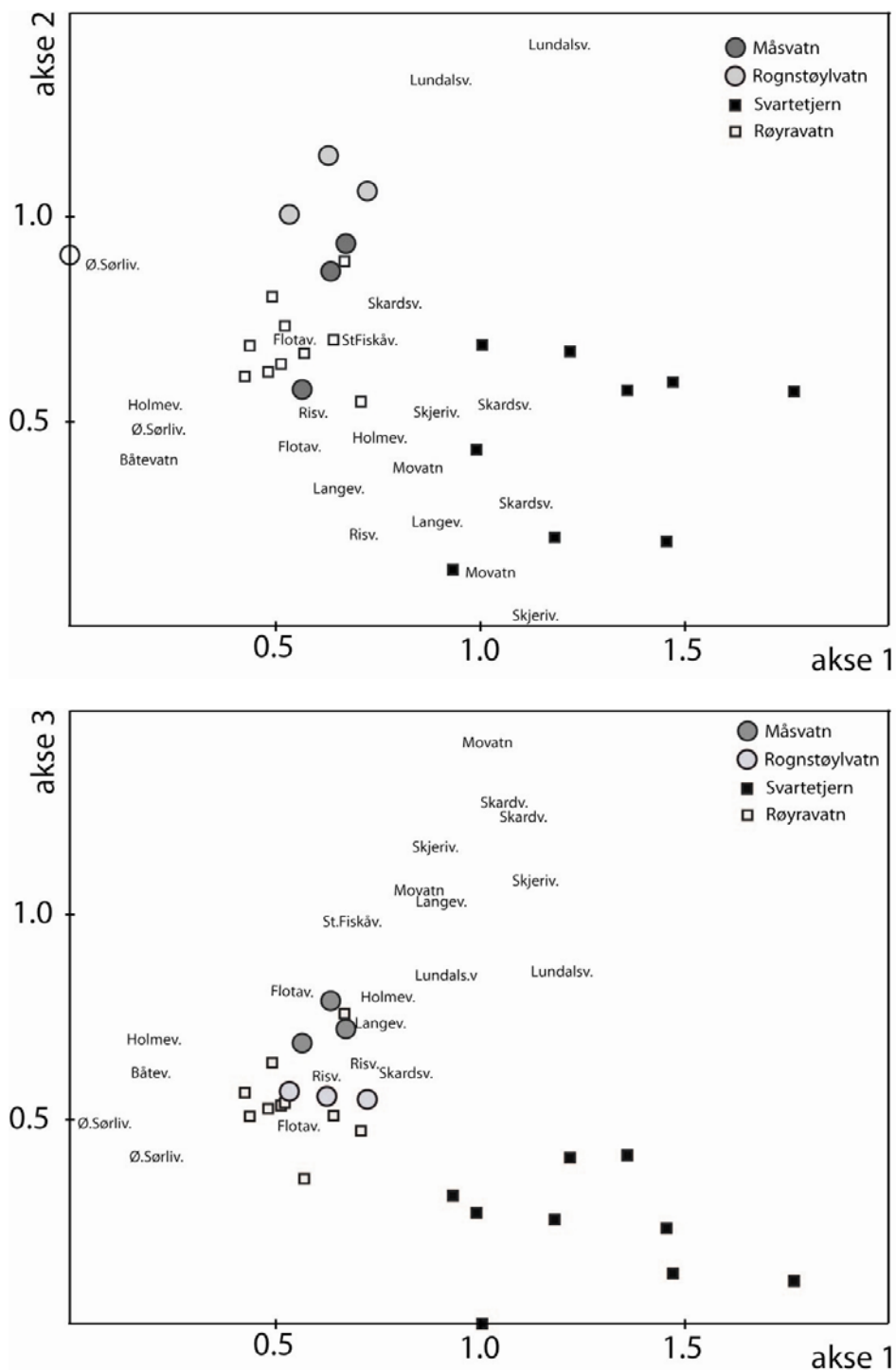
Figur 22. Krepssdyrsamfunnet i hhv. Rognestøylsvatn og Måsvatn sammenlignet med andre overvåkingslokaliteter av tilsvarende vann typer på Vestlandet og i Midt-Norge (forsuringsregion VI-VIII) basert på DCA analyser (CANOCO vers. 4.5). Innsjøer (og prøver) som viser stor likhet i krepssdyrfaunaen vil plasseres nær hverandre i diagrammet mens innsjøer (og prøver) som er mer forskjellige plasseres lengre fra hverandre. Øverste figur, akse 1 og 2, Nederste figur: akse 1 og 3. Røyrvatn og Svartetjern, to overvåkingslokaliteter med årlige undersøkelser, er angitt med symboler; de øvrige kun med navn. Analysene er basert på årlige artslistene der hver art er angitt med relativ forekomst gruppert i tre dominansklasser (1: <1 %, 2: 1-10 %, 3: >10 % av totalt antall småkreps i prøven). De fire første aksene forklarer totalt 32,4 % (hhv. 12,5, 10,1, 6,4 og 3,6 %) av totalvariasjonen i materialet.
