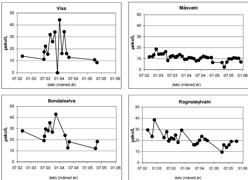
Figur 9. Klorid og ikke-marin sulfat i de fire undersøkte lokalitetene.
