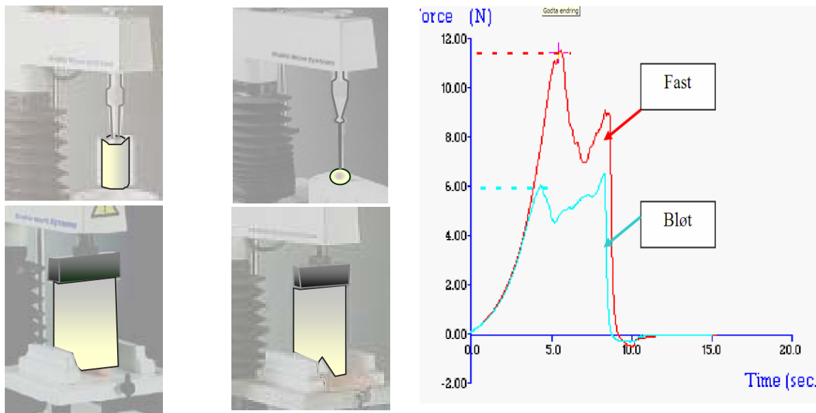
Figur 2 Eksempler på utstyr som benyttes ved instrumentelle teksturmålinger (venstre, Sigurgisladottir m.fl, 1999), og resultat fra teksturmåling av laks med fast og bløt tekstur (målt ved bruk av sylindere på fersk laks) (høyre, Mørkøre og Rørå 1999).
