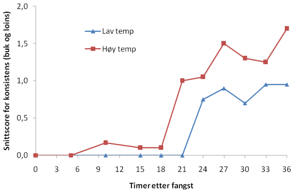
Figur 13 Konsistens (snittscore buk og loins), vurdert etter sløyting av torsk som var lagret usløydt inn til 36 timer etter fangst, ved lav og høy temperatur. Karakter 0 = fast naturlig konsistens, karakter 2 = bløt konsistens, n = 5 .
