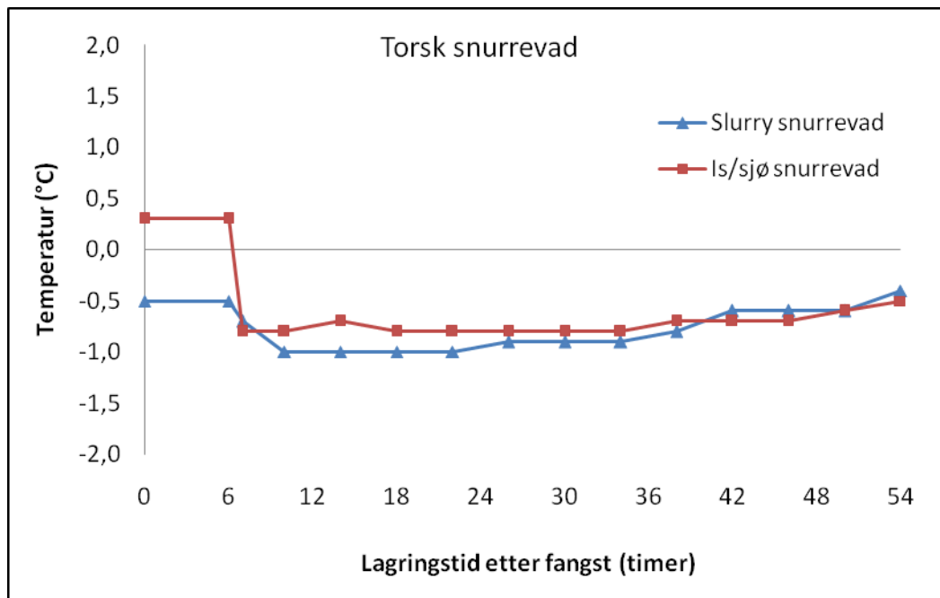
Figur 2 Temperatur fra fangst til sløyning i torsk fisket med snurrevad , under lagring usløydd i konteiner med slush-is (slurry) eller blanding av is/sjøvann, om bord på båten og på land.
