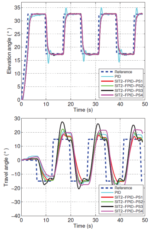
Fig. 7. Respuesta transitoria de un controlador difuso SIT2-FPID. La imagen es tomada del artículo Design and Experimental Validation of Single Input Type-2 Fuzzy PID Controllers as Applied to 3 DOF Helicopter Testbed [16]
