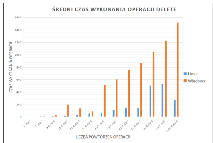
Rys. 4. Średni czas wykonania operacji DELETE
