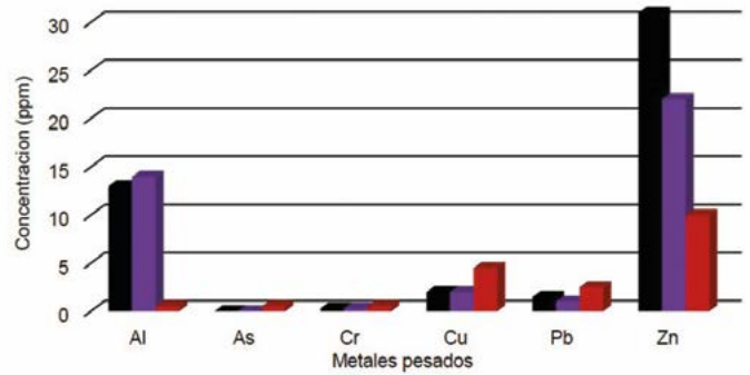
Figura 3. Concentración de metales pesados en muestras de suelo en los predios “La Finca” en Villa Guerrero (barra negra), “La Fábrica” en Tenancingo (barra morada), Limite Permisible (barra roja). Al: aluminio, As: arsénico, Cr: cromo, Cu: cobre, Pb: plomo, Zn: zinc.
