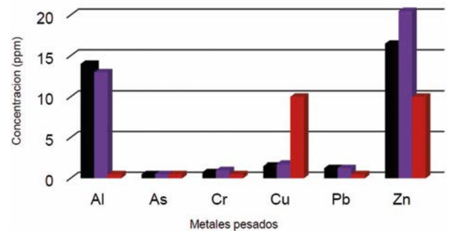
Figura 5. Concentración de metales pesados en muestras de fruto de fresa ( Fragaria xananassa Duch. var. festival) en los predios “La Finca” en Villa Guerrero (barra negra), “La Fábrica” en Tenancingo (barra morada), Limite Permisible (barra roja). Al: aluminio, As: arsénico, Cr: cromo, Cu: cobre, Pb: plomo, Zn: zinc.
