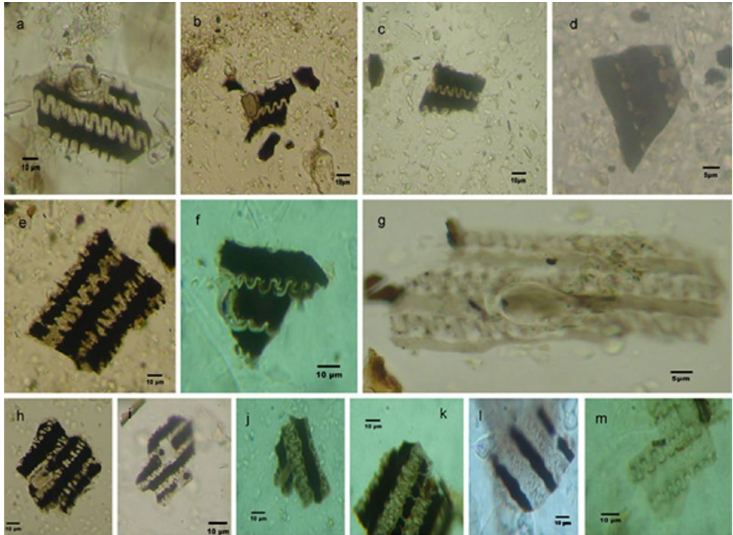
Figura 6. Láminas silíceas de gluma tipo Titicum sp. del Nivel II del Sondeo 2 de CH25. Algunas presentan restos de materia carbonosa adherida (a-c, e, f, h, i), y marcas de corte rectas (a, c, e, j) y curvas (b, d, e, i, j). También se pueden observar distintos grados de alteraciones y pérdida de materia orgánica adherida (e, g-m).
