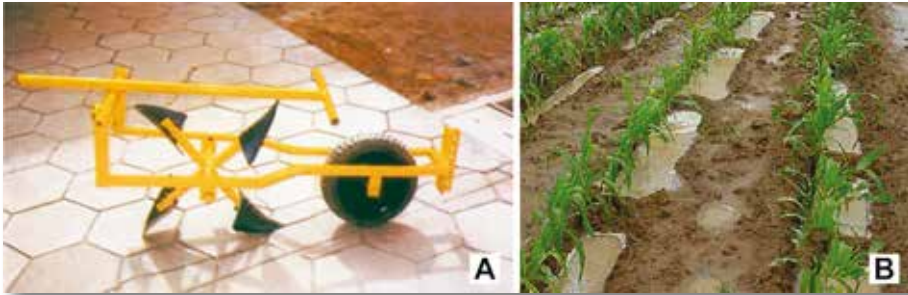
Figura 5. Barrador de sulcos (A) e barramento de sulcos em plantio de milho ( Zea mays ) (B).
