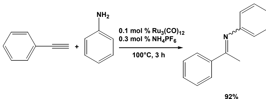
Schema 3. \text{Ru}_3(\text{CO})_{12} -katalysierte intermolekulare Hydroaminierung von Phenylacetylen.
