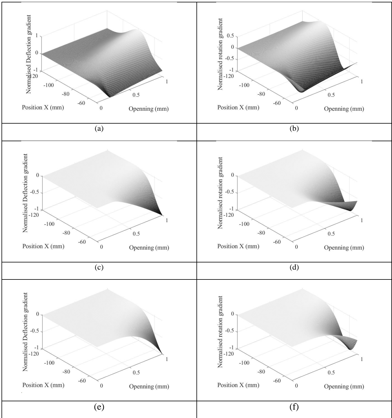
Figure 8 : Fonctions des sensibilités obtenue par CIN respectivement en déplacement et rotation : (a) et (b) Sensibilité au module ; (c) et (d) Sensibilité à la contrainte maximale ; (e) et (f) Sensibilité au taux de restitution d'énergie critique.
