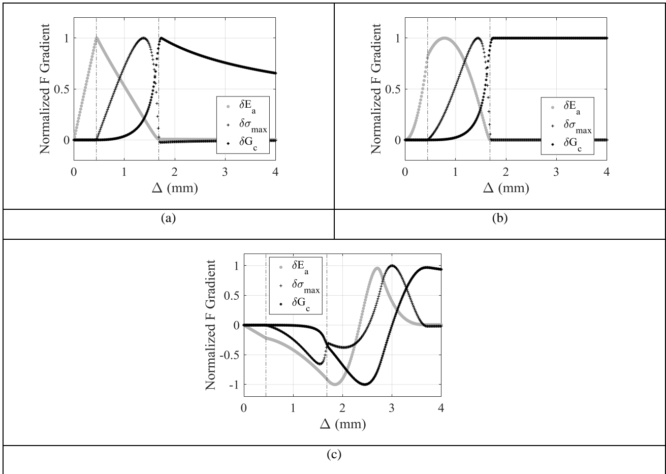
Figure 7 : Fonctions de sensibilités des paramètres : (a) Force-déplacement ; (b) Intégrale J ; (c) Jauge.
