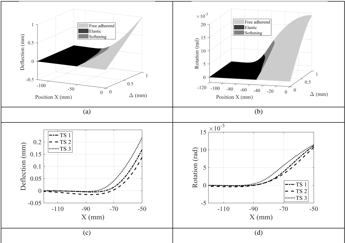
Figure 6 : Corrélation d'images numériques respectivement en déplacement et rotation : (a) et (b) mise en évidence des différentes phases de l'essai ; (c) et (d) influence de la loi TS utilisée
