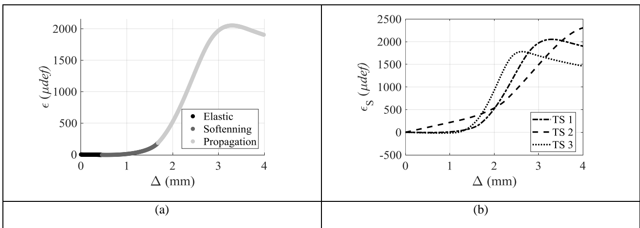
Figure 5 : Evolution du signal d'une jauge en fonction de l'ouverture en pointe de fissure : (a) mise en évidence des différentes phases de l'essai ; (b) influence de la loi TS utilisée
