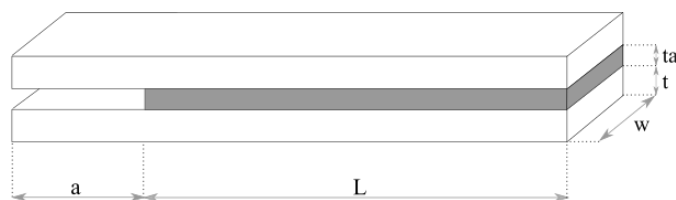
Figure 1 : Longueurs caractéristiques de l'éprouvette DCB
