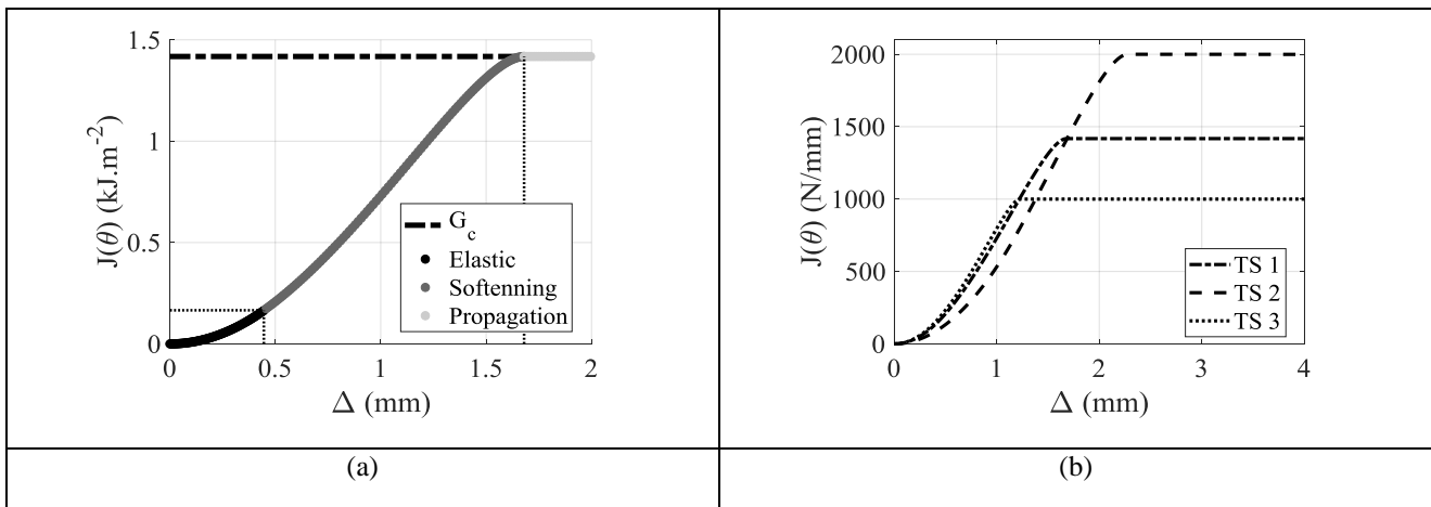
Figure 4 Evolution de l'intégrale J en fonction de l'ouverture en pointe de fissure : (a) mise en évidence des différentes phases de l'essai ; (b) influence de la loi TS utilisée
