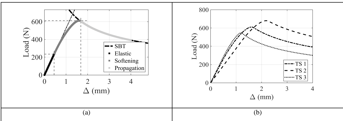
Figure 3 : Courbes force-déplacement : (a) mise en évidence des différentes phases de l'essai ; (b) influence de la loi TS utilisée
