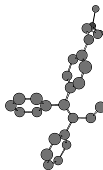
E - Tamoksifen
