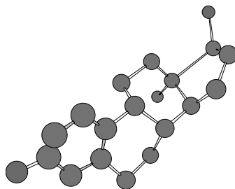
17 \beta -estradiol
