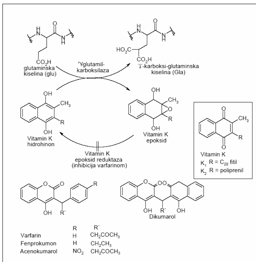
Slika 3 Shema inaktivacije \gamma -glutamylkarboksilaze u prisustvu antagonista K vitamina
