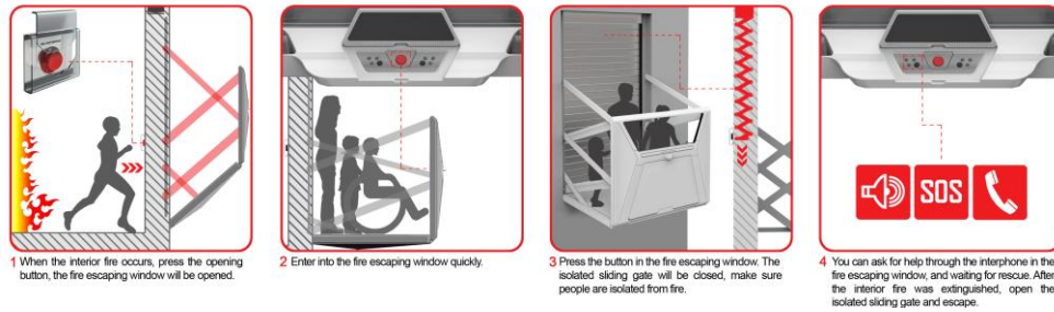
图 6 火灾救生窗的使用流程
