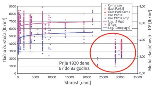
Slika 7. Razvoj tlačne čvrstoće (plava linija) i modula elastičnosti (ružičasta linija) betona koji nisu degradirali [17]; 1,0 \text{ lb/in}^2 = 0,006895 \text{ N/mm}^2 \text{ (MPa)} ; 1,0 \text{ MPa} = 145,04 \text{ lb/in}^2
