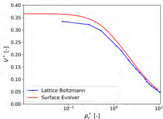
Figure 8.9: Volume en fonction de la pression capillaire pour les sphères en contact dans des conditions de drainage. Comparaison entre LBM et les résultats pour SE extraits de Wang et al. (2017).
