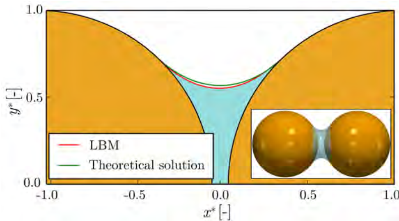
Figure 8.26: Perfils de ponts capil·lars superposats obtinguts numèricament i analíticament per una pressió capil·lar de p_c^* = 0.6 .
