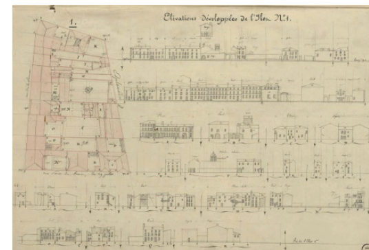
Fig. 10 - Plan-Relief de Toul. Magasins à Fourrages. 1/600. 1848. [Relevés préparatoires du plan-relief de Toul. Paris, musée des Plans-Reliefs, Archives]
