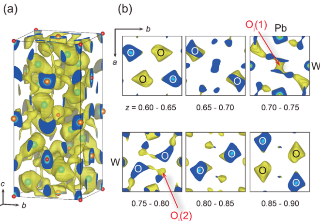
Rietveld解析とMEM解析により求めた核密度分布。黄色色の分布が酸素イオンの経路に相当する。右の⑥湯の図はz軸の各位置でスライスした断面図。
