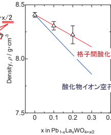
Pb 1-x La x WO 4+x/2 の粉末密度測定結果。
