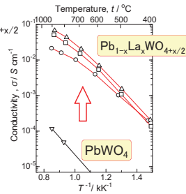
Pb 1-x La x WO 4+x/2 の導電率のアレニウスプロット。 ∇: x = 0, ○: x = 0.1, △: x = 0.2, □: x = 0.3.
