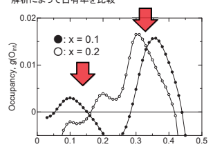
(0 0 z)に格子間酸化物イオンを仮定したときの占有率
