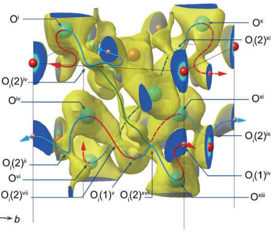
3次元的な導電パスの拡大図。
