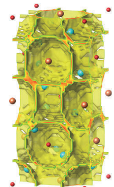
静電的相互作用のみから予想される導電パス。
