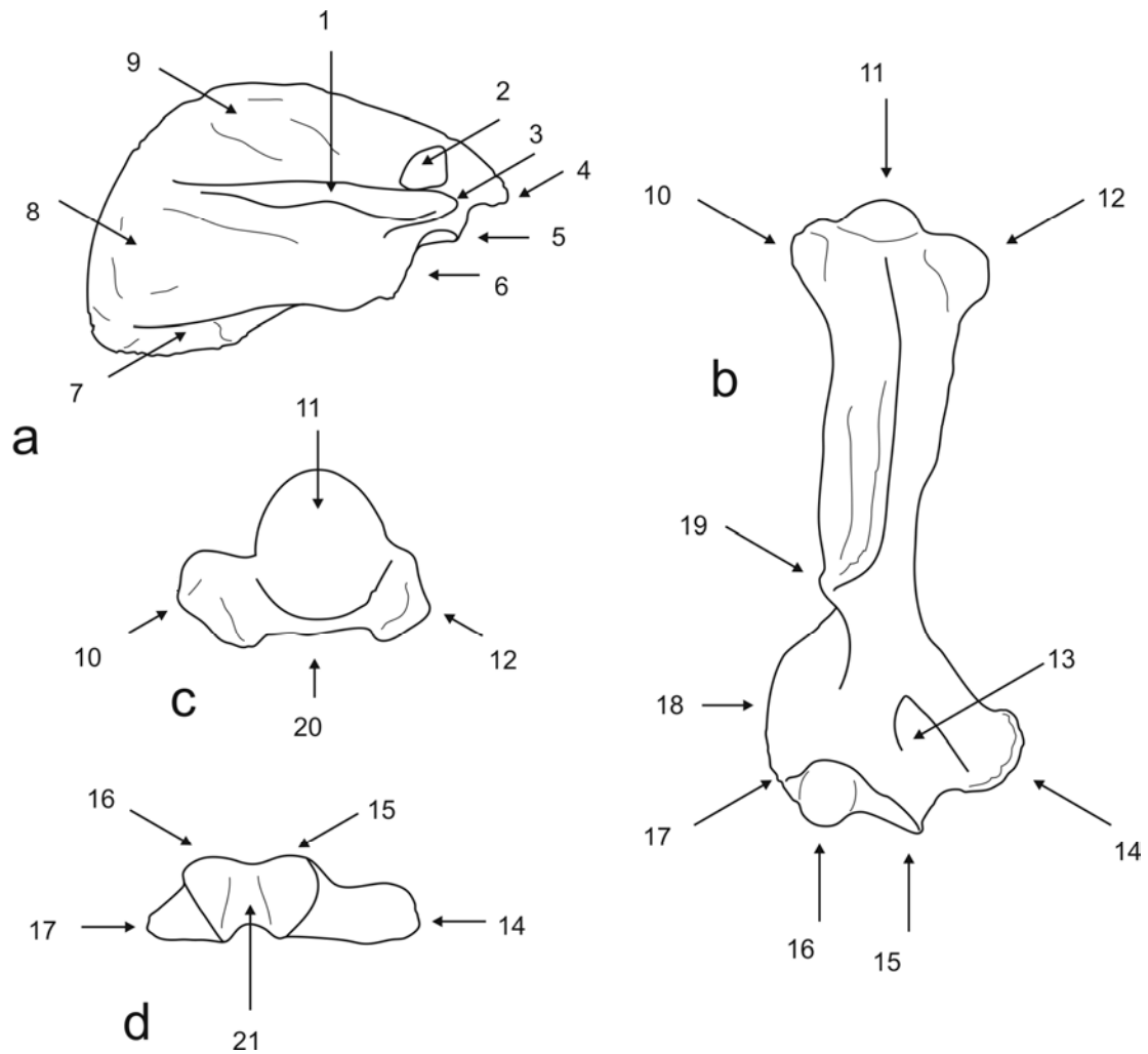
Figura 5.1. Accidentes anatómicos de importancia en esta Tesis, representados en un espécimen generalizado de perezoso santacrucense: a- escápula derecha, vista lateral (extremo ventral hacia la derecha); b- húmero derecho, vista anterior; c- húmero derecho, vista proximal (la cara anterior hacia abajo); d- húmero derecho, vista distal (cara anterior hacia arriba). 1- espina escapular, 2- foramen escapulo-coracoideo; 3- acromion; 4- proceso coracoideo; 5- tubérculo supraglenoideo, 6- fosa glenoidea escapular; 7- fosa postescapular; 8- fosa infraespinosa; 9- fosa supraespinosa; 10- tuberosidad mayor (lateral) del húmero; 11- cabeza humeral; 12- tuberosidad menor (medial) del húmero; 13- canal entepicondilar; 14- entepicóndilo; 15- tróclea humeral; 16- capítulo humeral; 17- ectepicóndilo; 18- cresta epicondilar, 19- plataforma deltopectoral; 20- surco bicipital.
