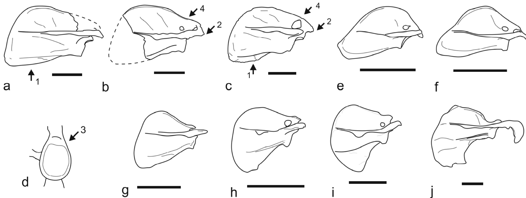
Fig. 6.1. Escápulas derechas en vista lateral. a- Hapalops MPM-PV 3412; b- Hapalops angustipalatus YPM-VPPU 15562; c- Eucholoeps fronto MPM-PV 3403; d- El mismo espécimen, fosa glenoidea en vista anterior; e- Bradypus variegatus AMNH 42838; f- Choloepus didactylus AMNH 35483; g- Cyclopes didactylus FMNH 81889; h- Tamandua mexicana AMNH 23565; i- Myrmecophaga tridactyla FMNH 26563; j- Priodontes maximus FMNH 25271. 1- fosa postescapular; 2 posición del arco coracoideo; 3 tubérculo supraglenoideo; 4- foramen coraco-escapular. Escala = 5cm (excepto en g-, escala = 2 cm.).
