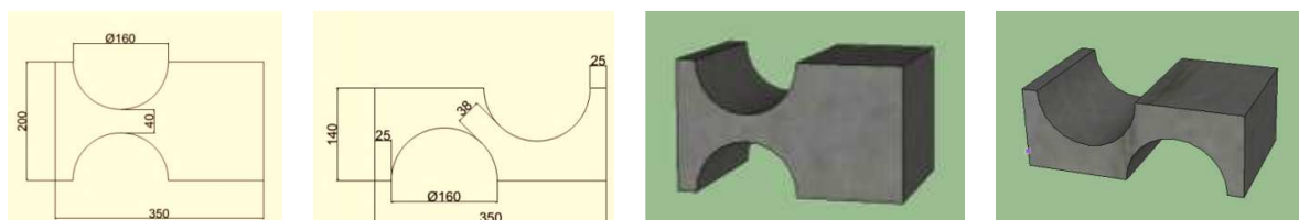
Figura 3: Plano y vista en 3D piezas
