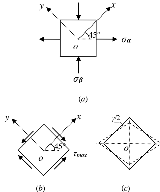
图 1 纯剪应力状态示意图
