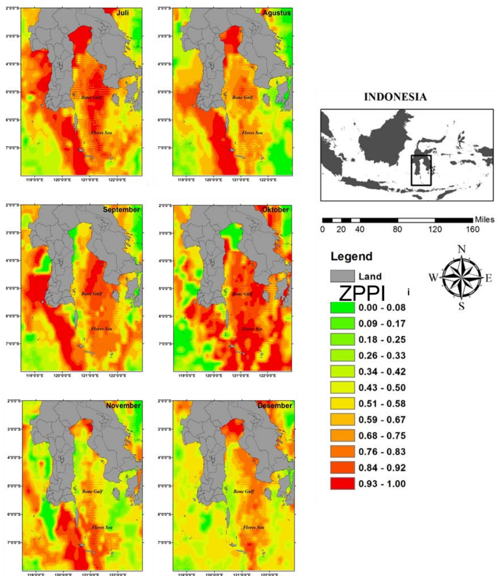
Gambar 4. Peta ZPPI Pelagis Besar pada Bulan Juli s.d Desember di Perairan Teluk Bone.
