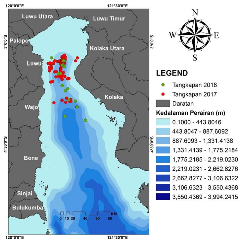
Gambar 1. Peta bathymetri (profil kedalaman) Perairan Teluk Bone yang dioverlay dengan Posisi Penangkapan ikan pelagis besar pada tahun 2017 dan 2018.
