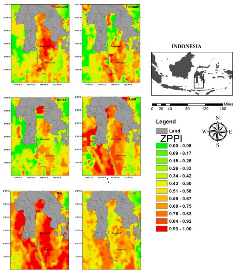
Gambar 3. Peta ZPPI Pelagis Besar pada Bulan Januari s.d Juni di Perairan Teluk Bone.
